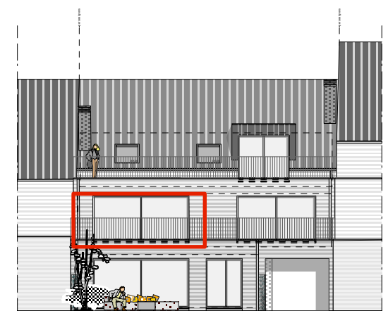
ACHTERGEVEL AANZICHT
