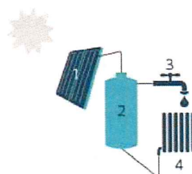
1. Zonnecollector | 2. Opslagvat zonneboiler | 3. Sanitair warm water | 4. Afgritelement voor ruimteverwarming (optioneel)
