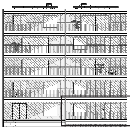
Noord gevel
