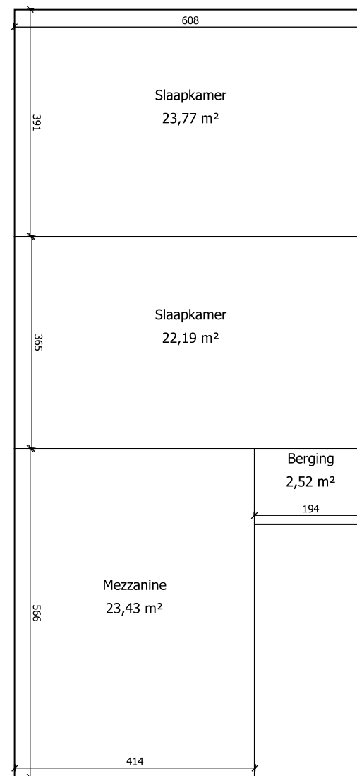
1ste verdieping
