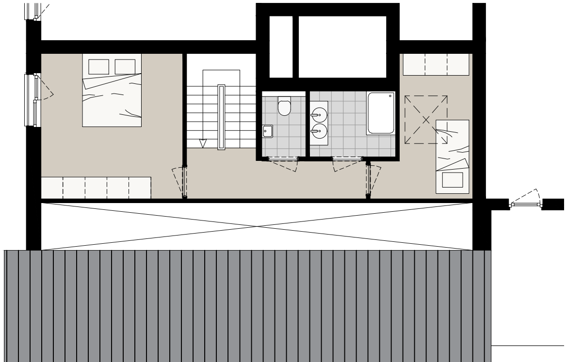
Niveau +2
