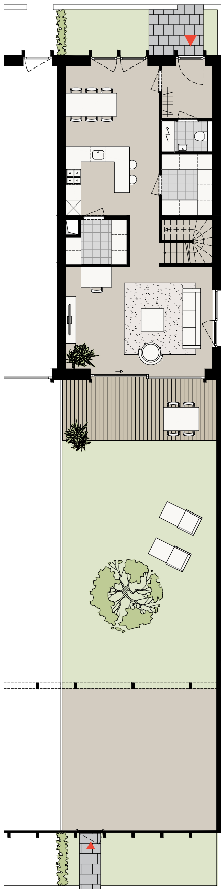
Gelijkvloers
