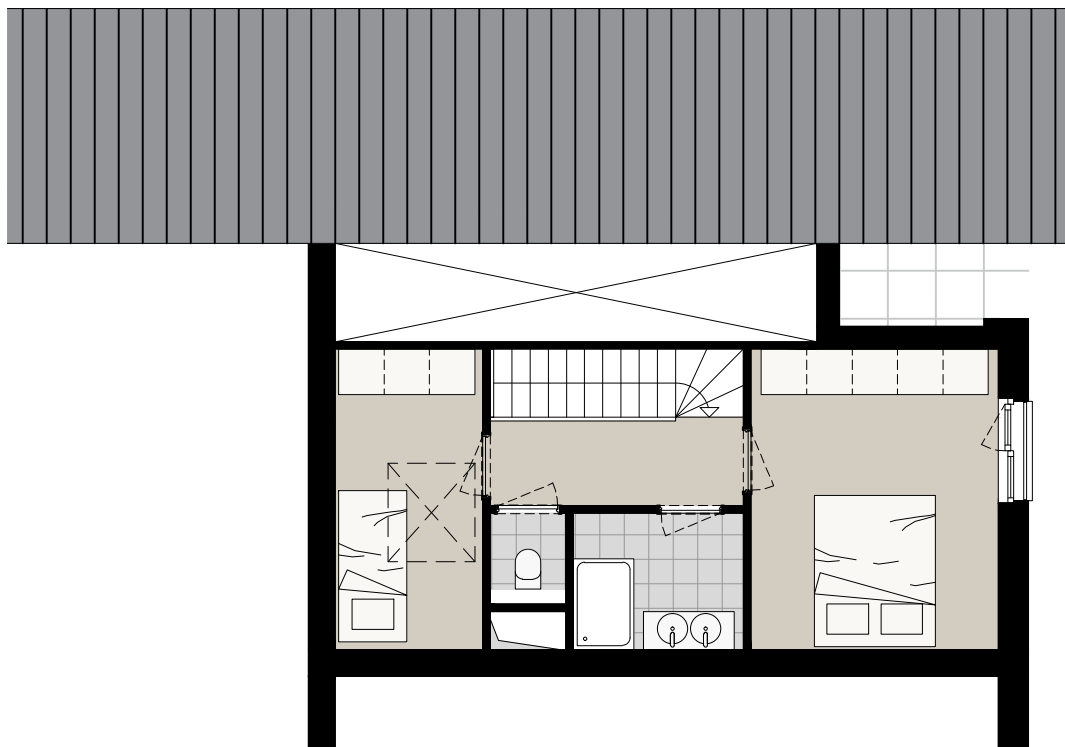
Niveau +2
