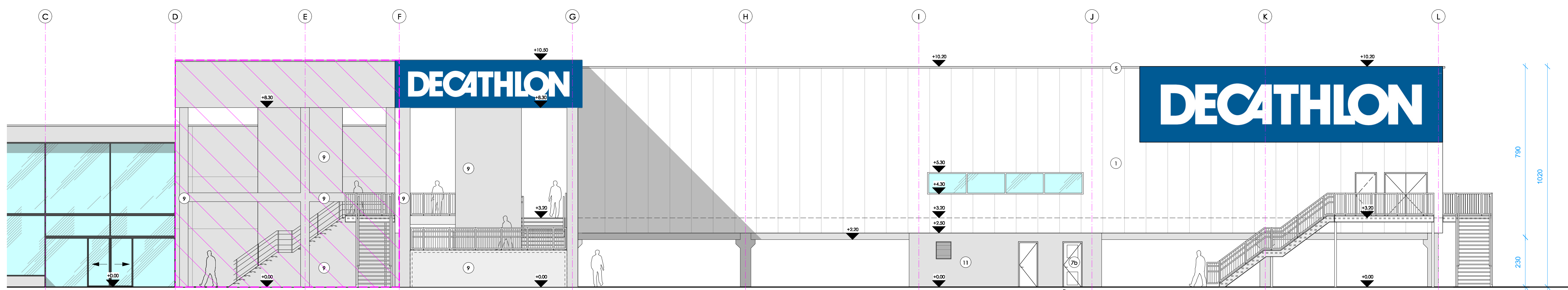
ZIJAAZICHT HANDELSRUIMTE 3 - PARKINGZIJDE schaal 1/100
