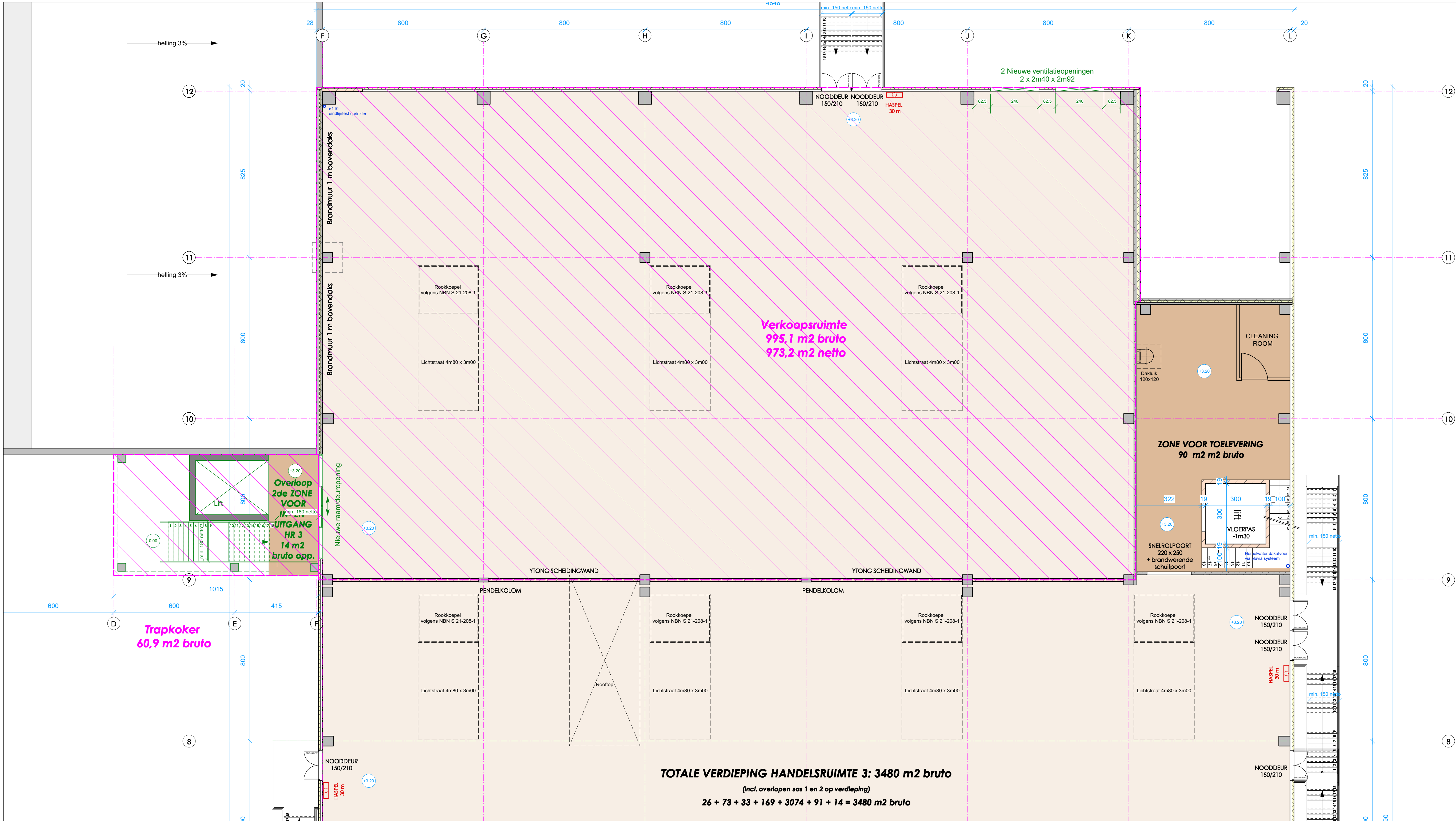
GRONDPLAN HANDELSRUIMTE 3: NIVEAU 1 schaal 1/100
