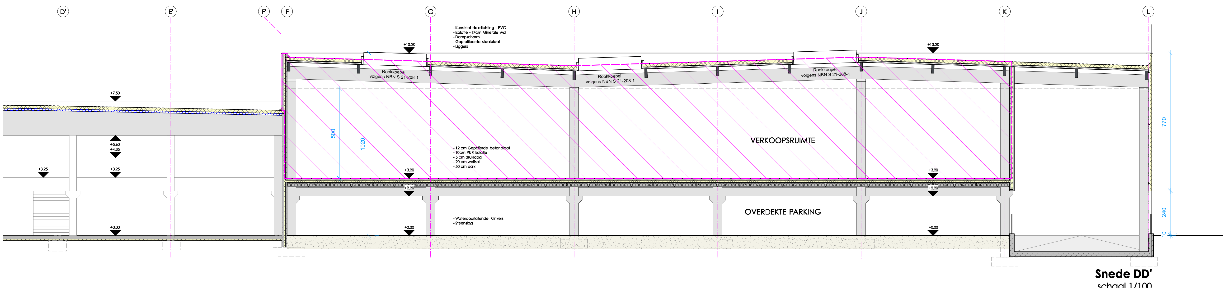
SneDE DD' schaal 1/100
