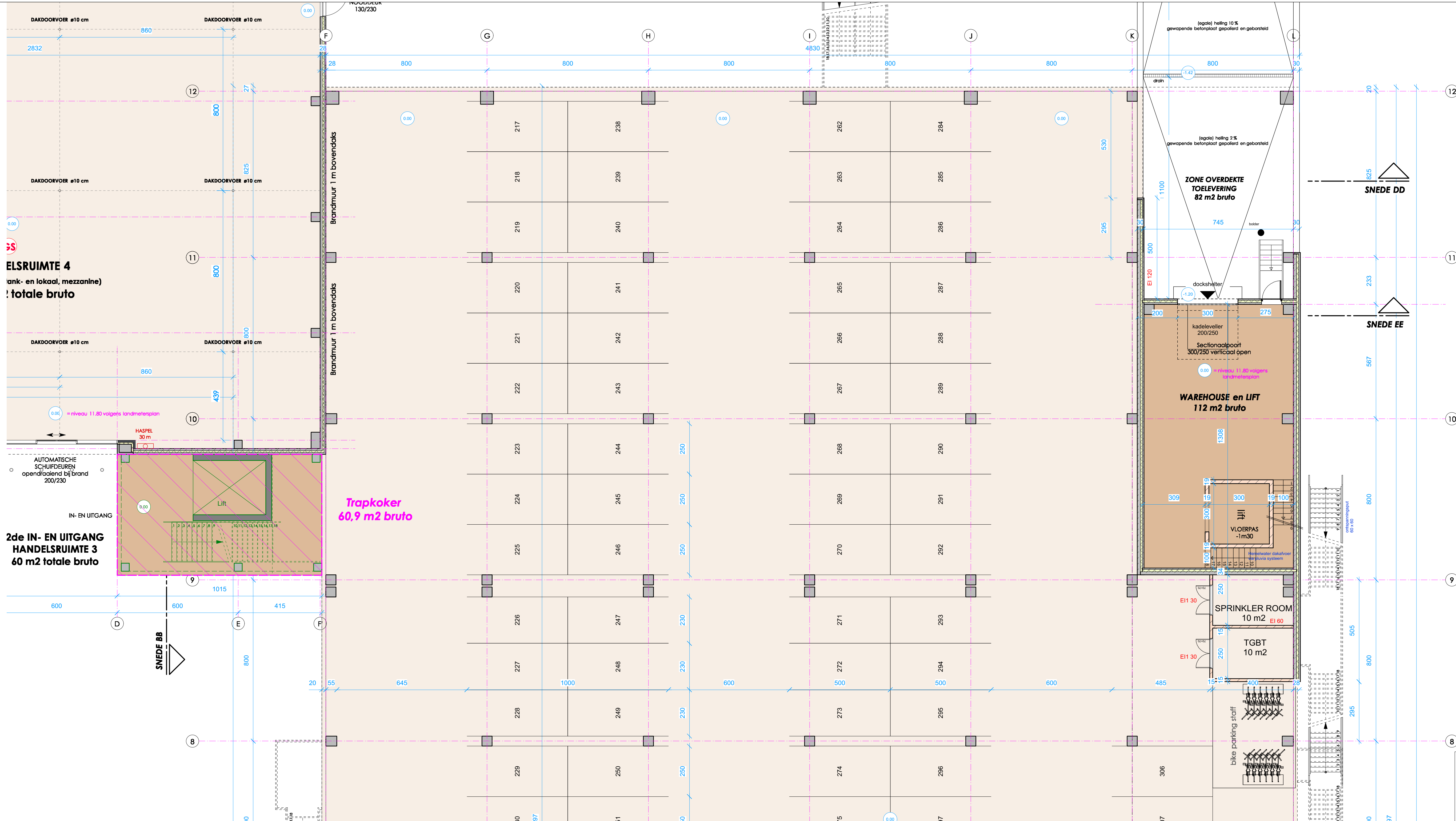
GRONDPLAN HANDELSRUIMTE 3: NIVEAU 0 schaal 1/100
