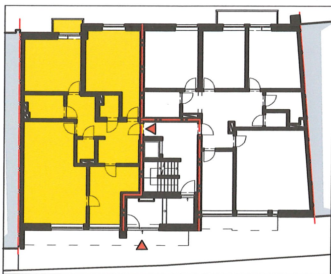
Plan de situation de l'appartement au rez
