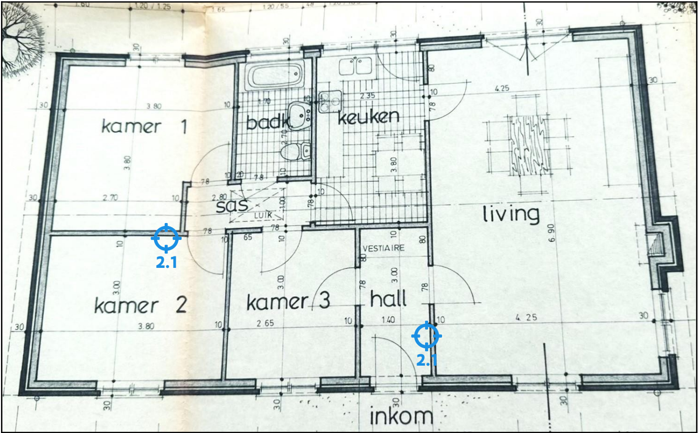
Legende van plan 1.2: Hoofdgebouw gelijkvloers
