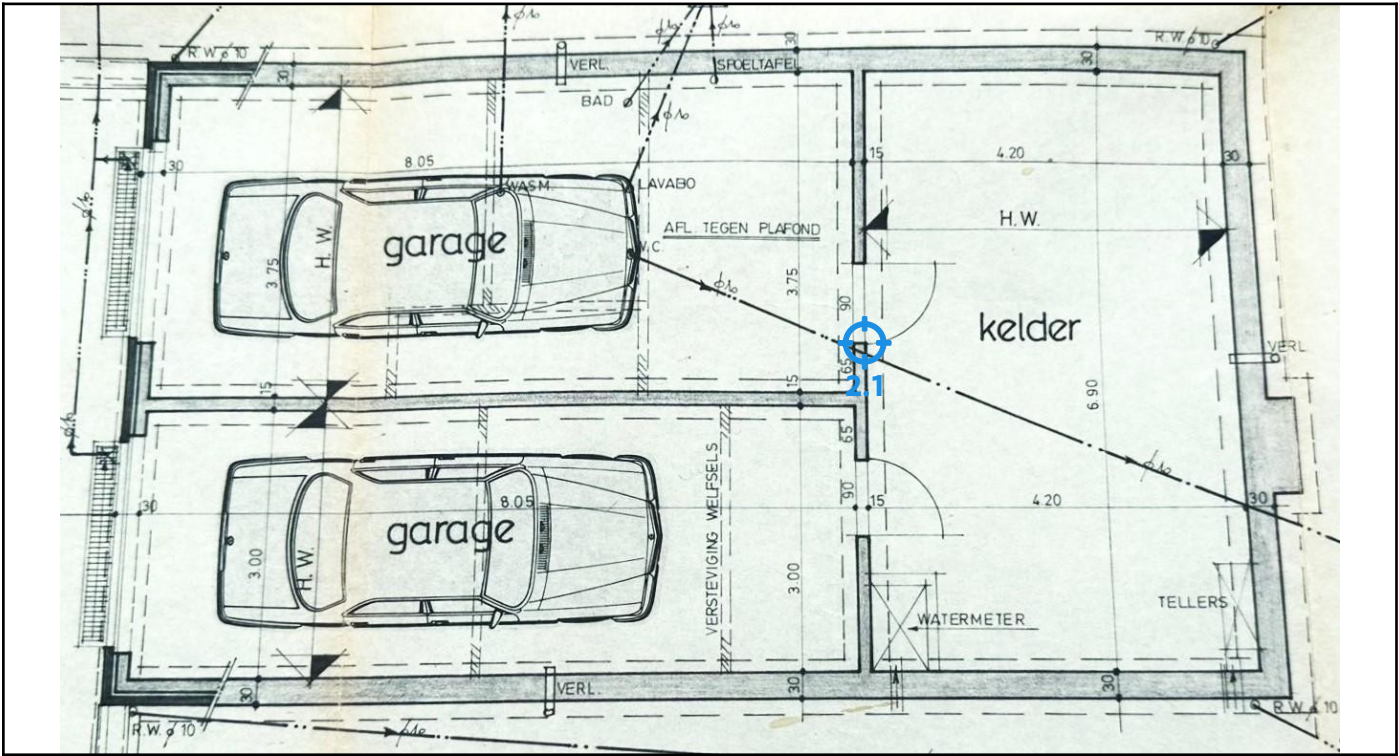
Legende van plan 1.1: Hoofdgebouw kelder
