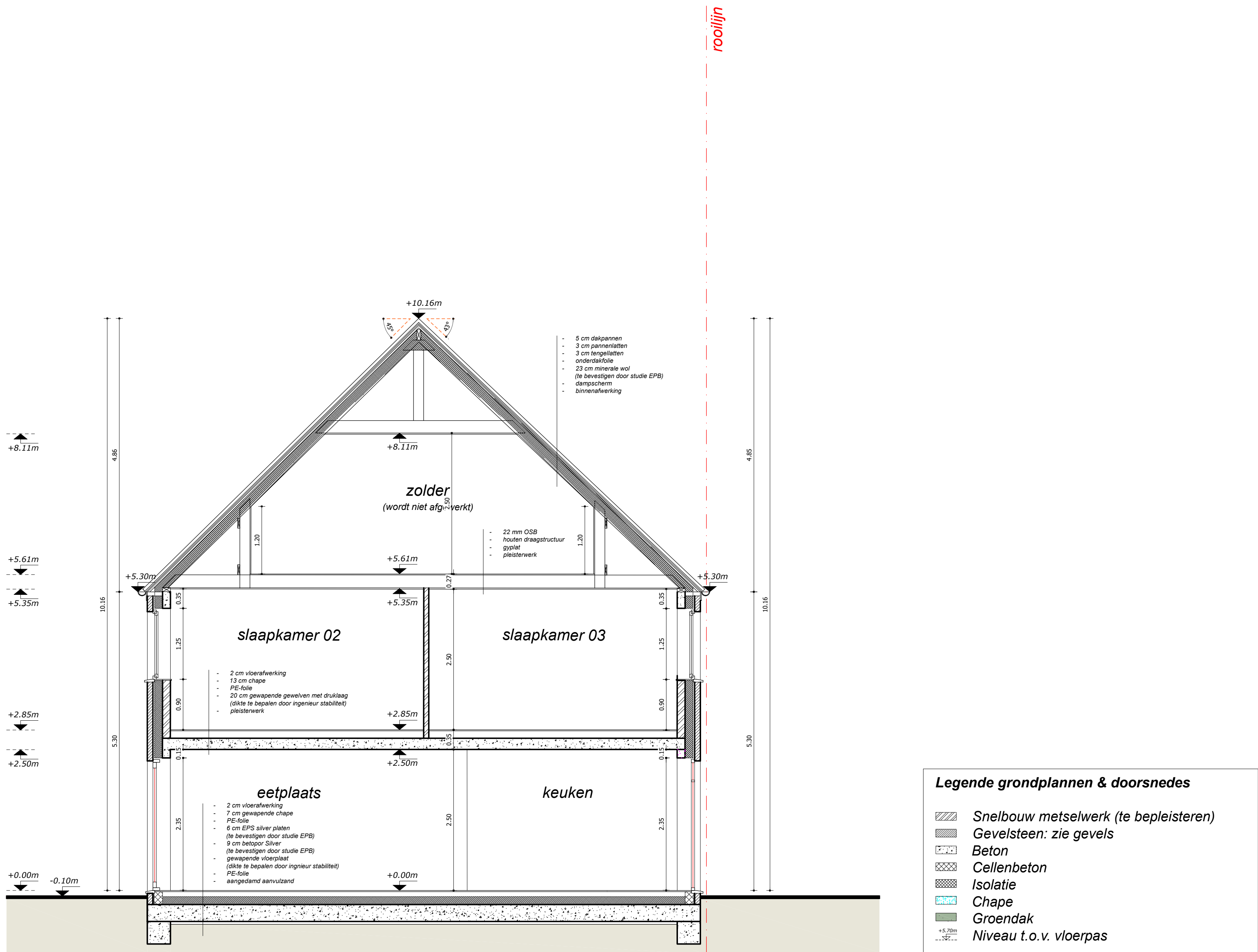
doorsnede CC' schaal 1:50 0 1 2 3 4 5
