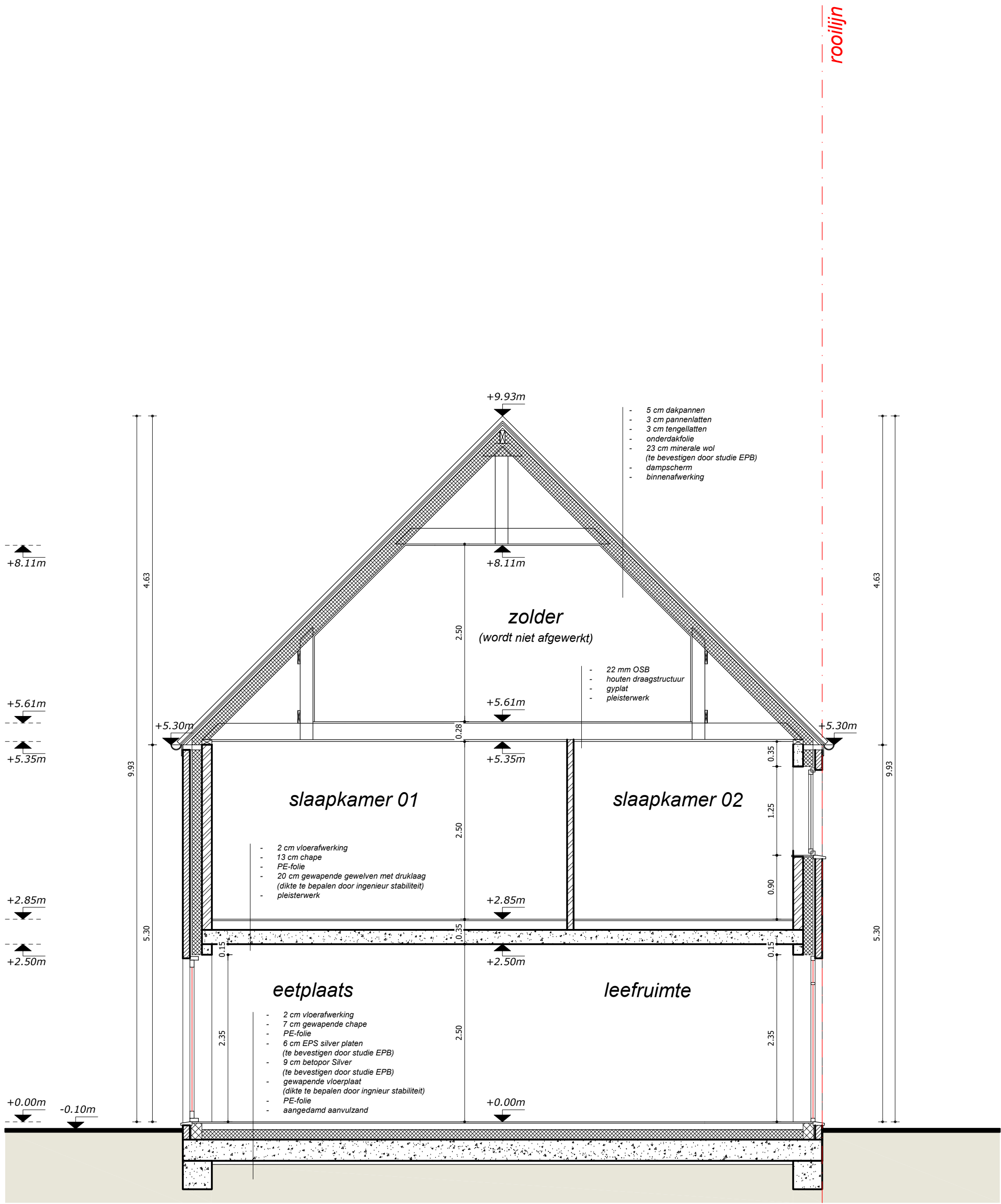
doorsnede EE' schaal 1:50
