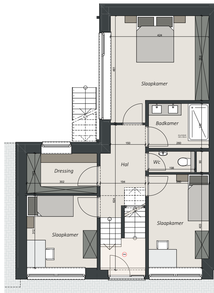
GELIJKVLOERS
