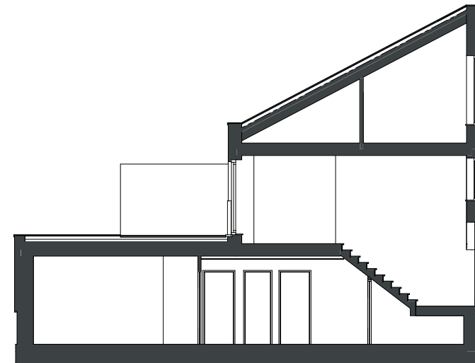
PRINCIPEDOORSNEDE
