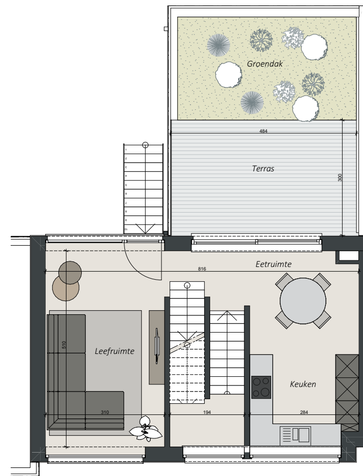
EERSTE VERDIEPING
