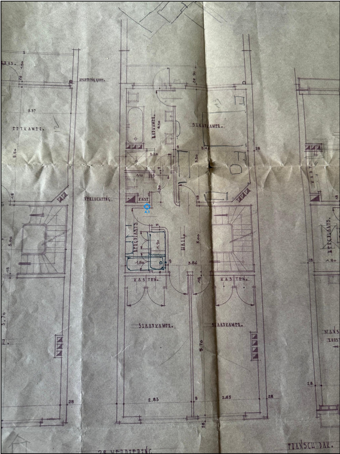
Legende van plan 1.4: 2de verdieping
