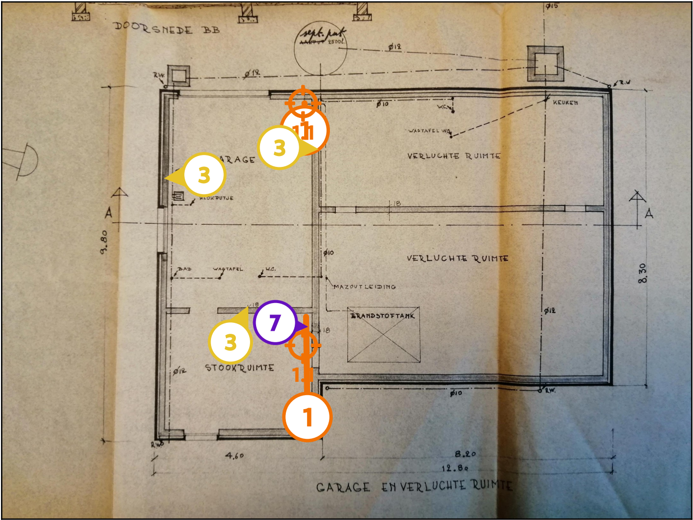
Legende van plan 1.1: grondplan fundering
