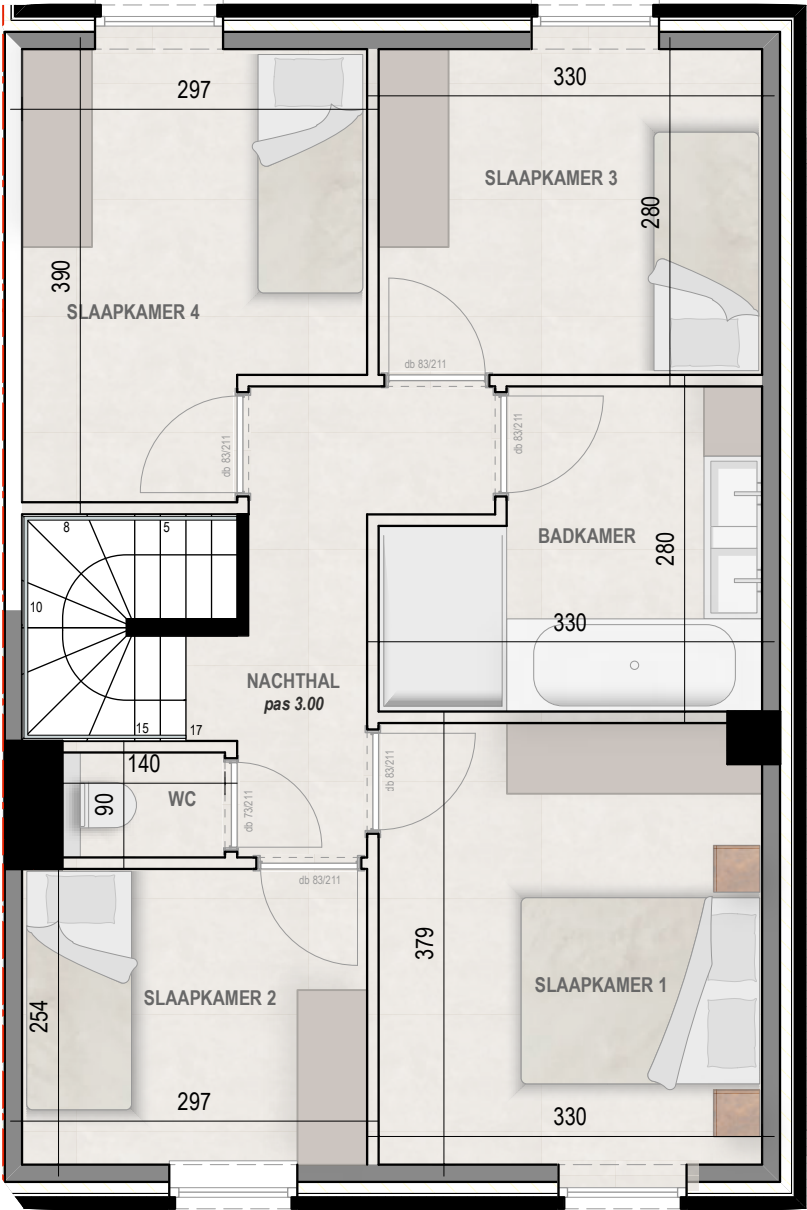
EERSTE VERDIEPING
