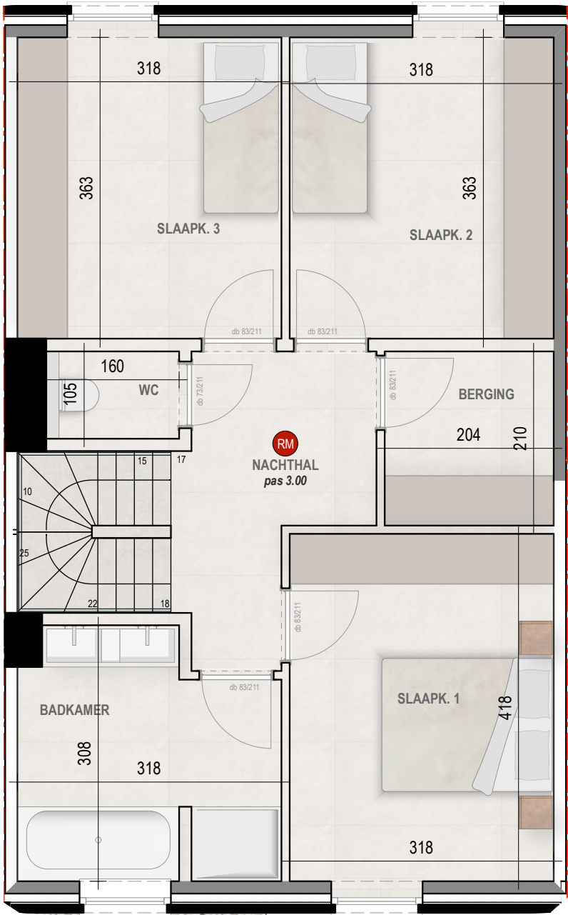
EERSTE VERDIEPING
