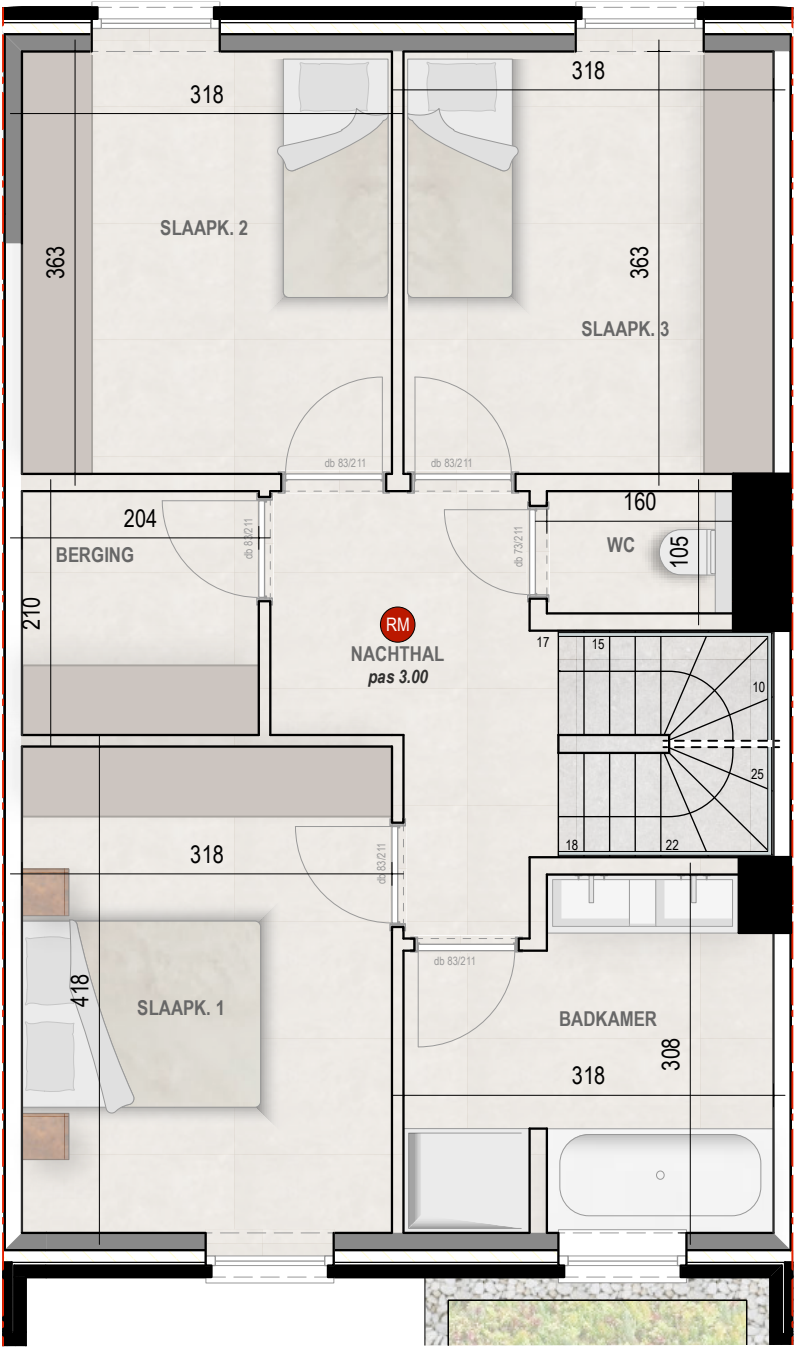
EERSTE VERDIEPING
