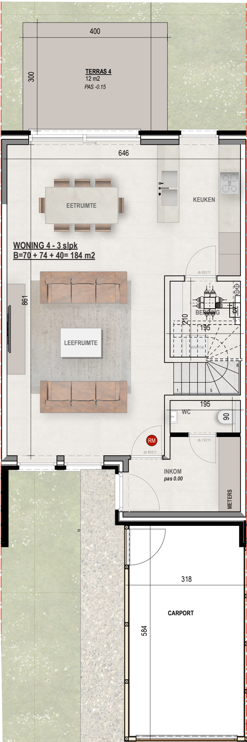
GELIJKVLOERS
