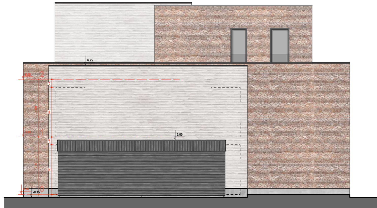
GEBOUW 1 - ZIJGEVEL - GEVEL 4 nieuwe toestand - schaal 1/100
