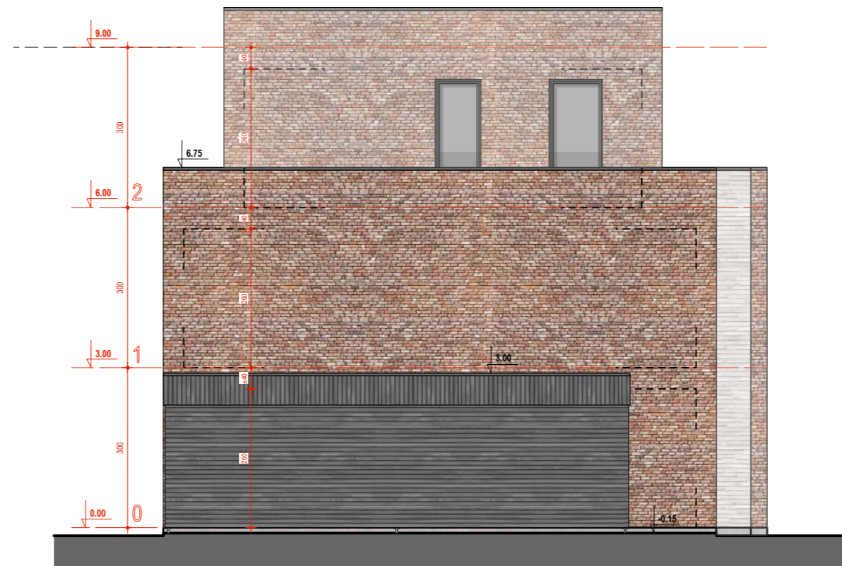
GEBOUW 2 - ZIJGEVEL - GEVEL 4 nieuwe toestand - schaal 1/100
