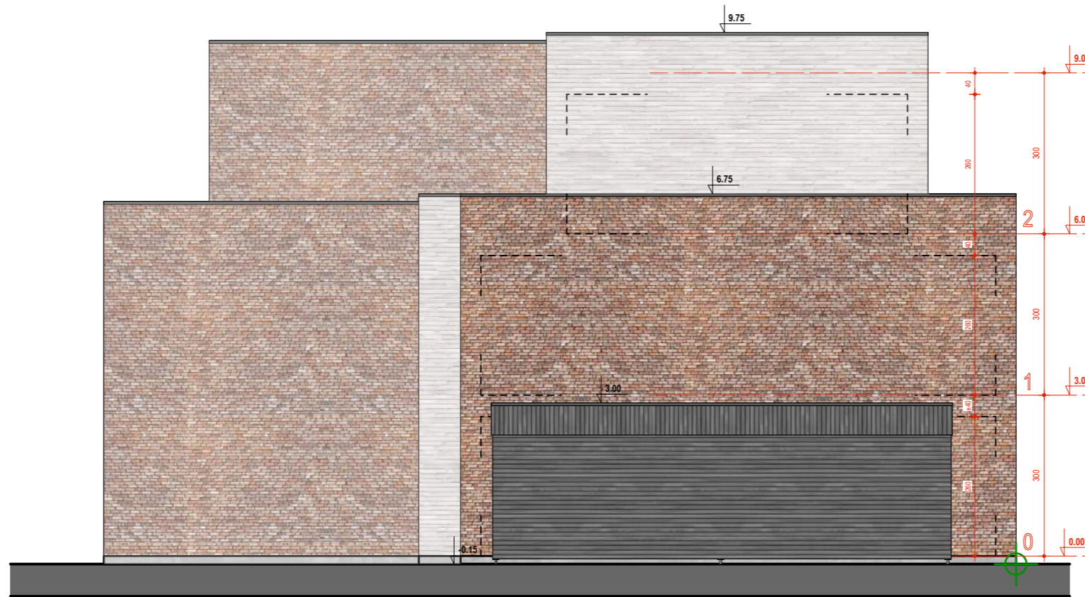
GEBOUW 1 - ZIJGEVEL - GEVEL 3 nieuwe toestand - schaal 1/100
