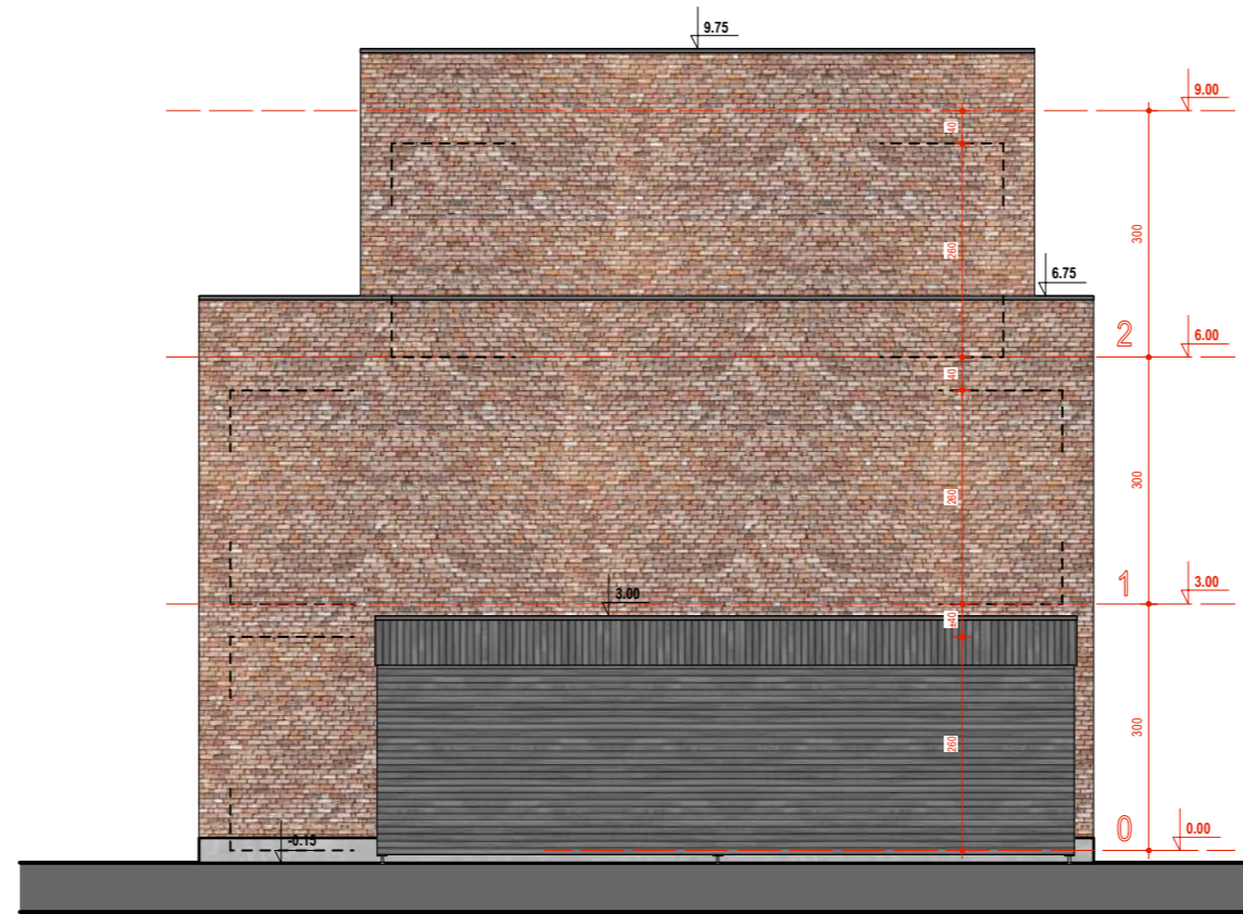
GEBOUW 2 - ZIJGEVEL - GEVEL 3 nieuwe toestand - schaal 1/100
