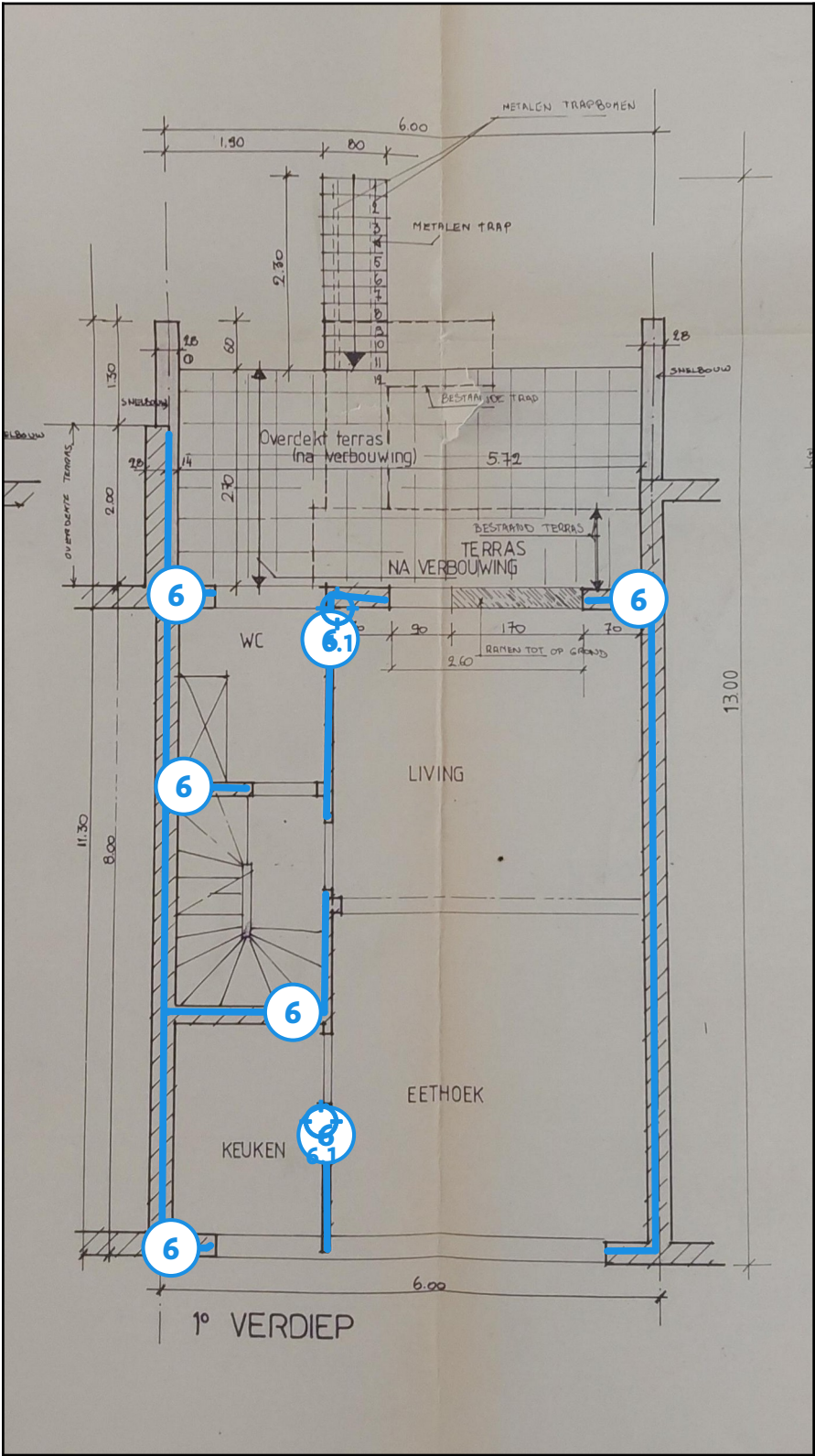
Legende van plan 1.5: Verdieping 1
