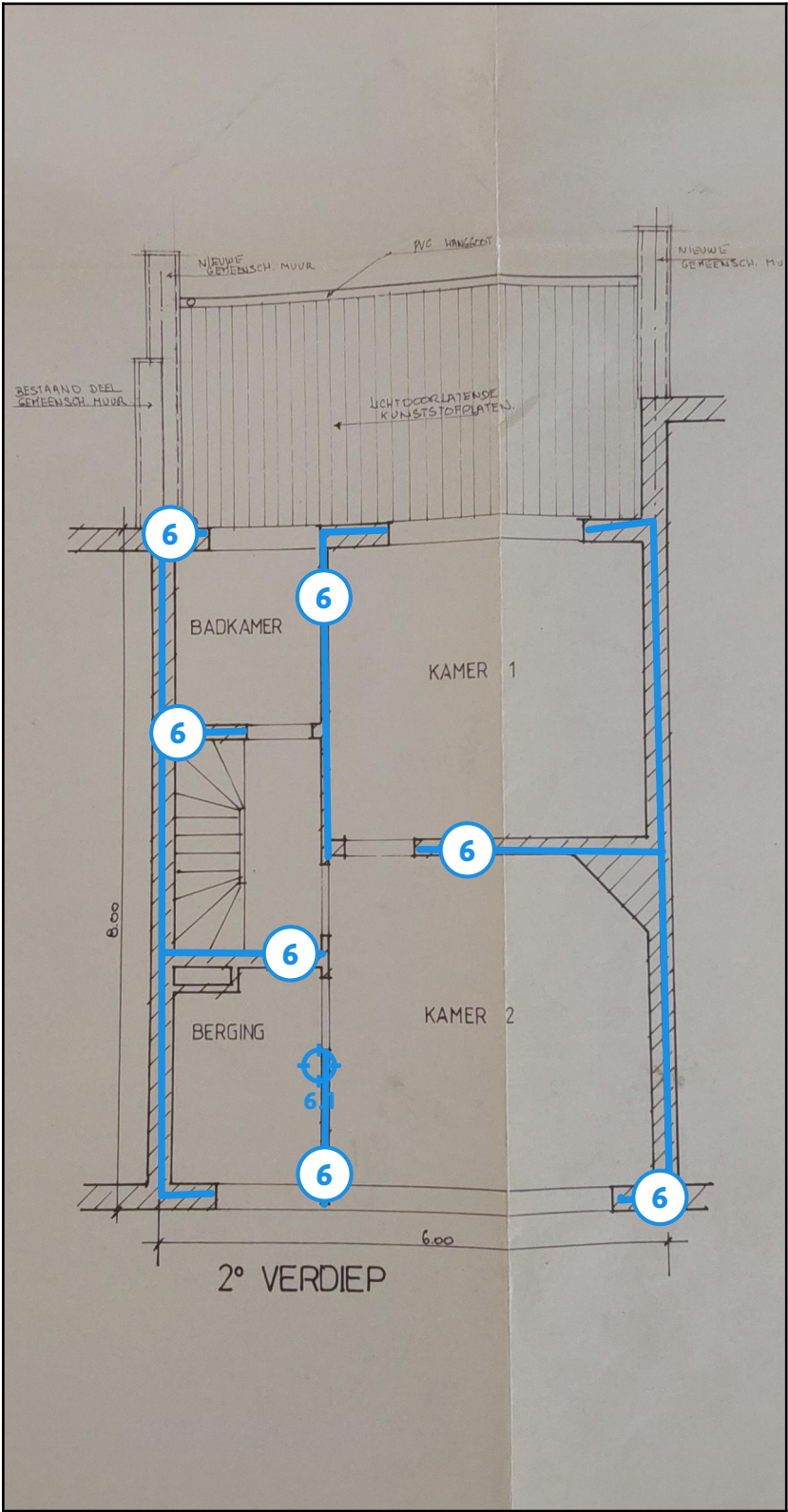
Legende van plan 1.8: Verdieping 2
