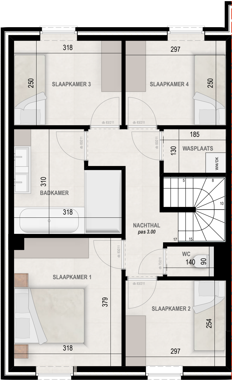
EERSTE VERDIEPING
