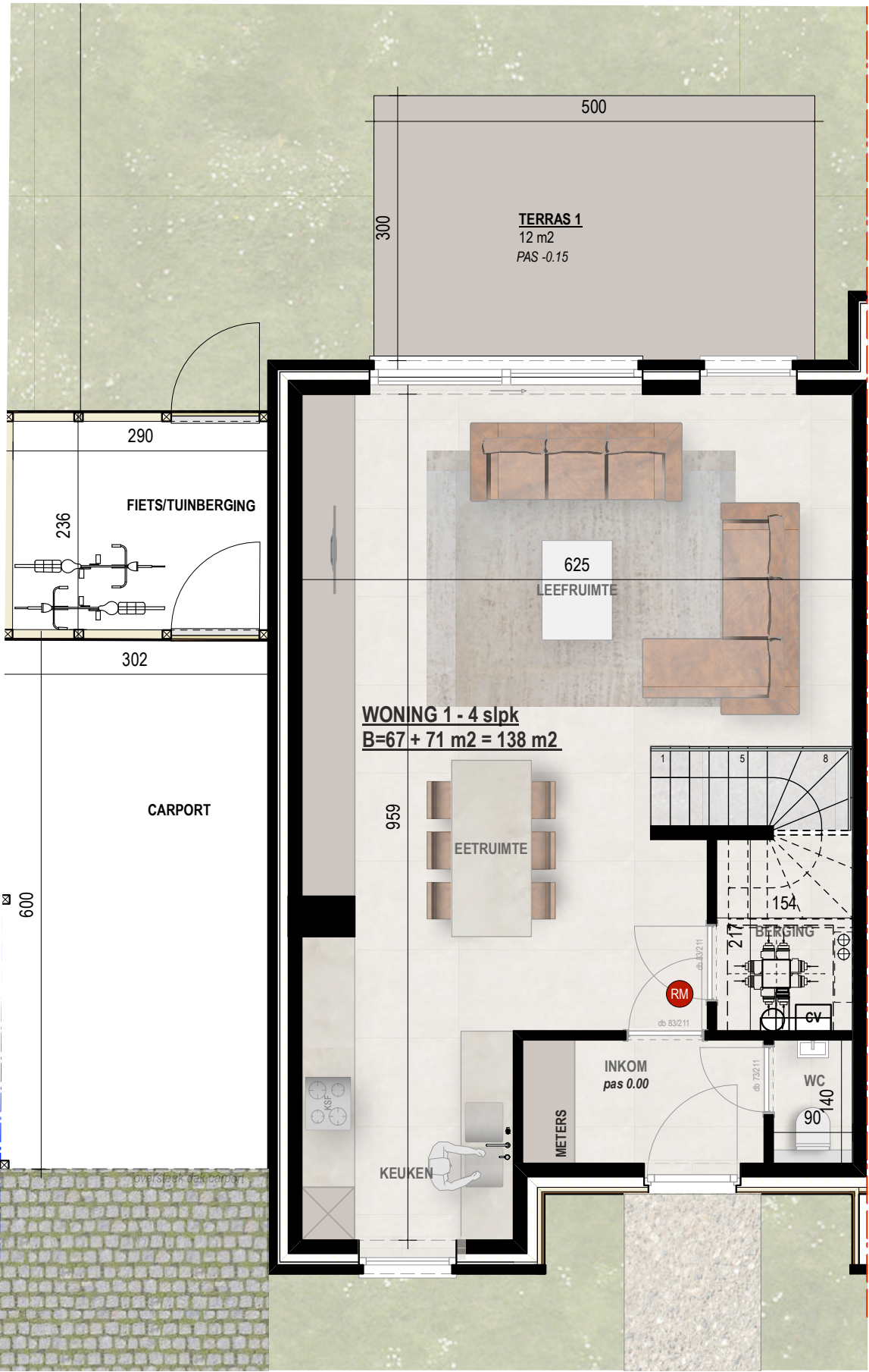
GELIJKVLOERS
