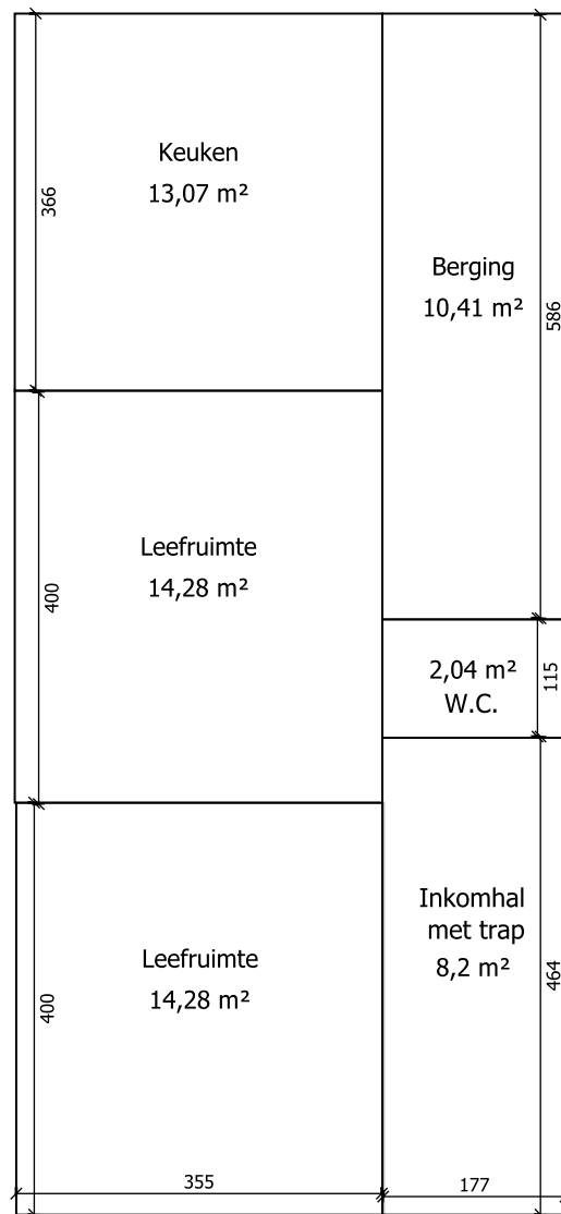
Gelijkvloers
