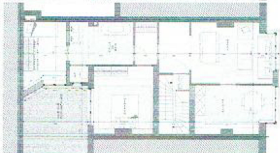
PLAN DU 3ème ETAGE 1:50 SITUATION PROJETEE
