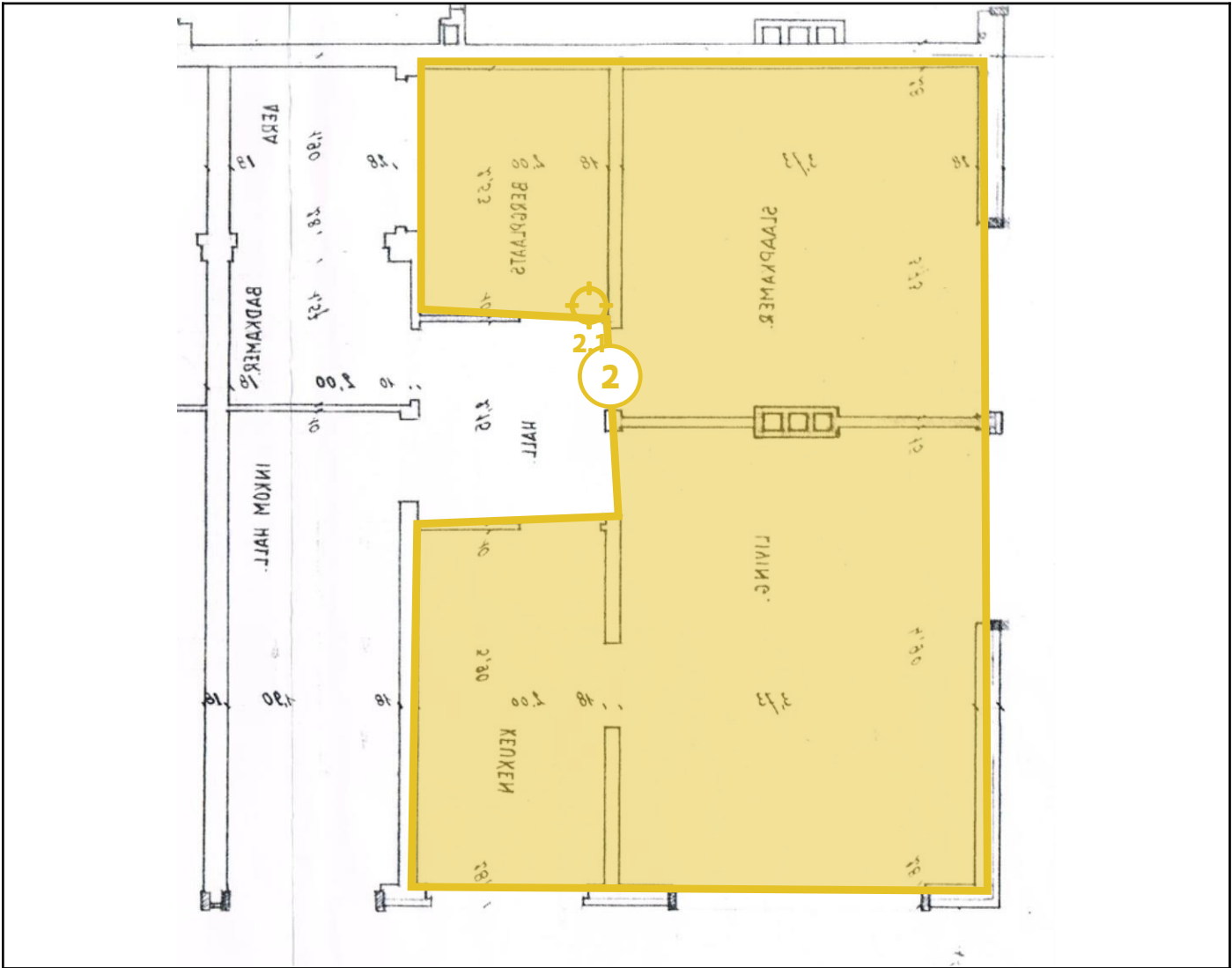
Legende van plan 1.4: Appartement 201
