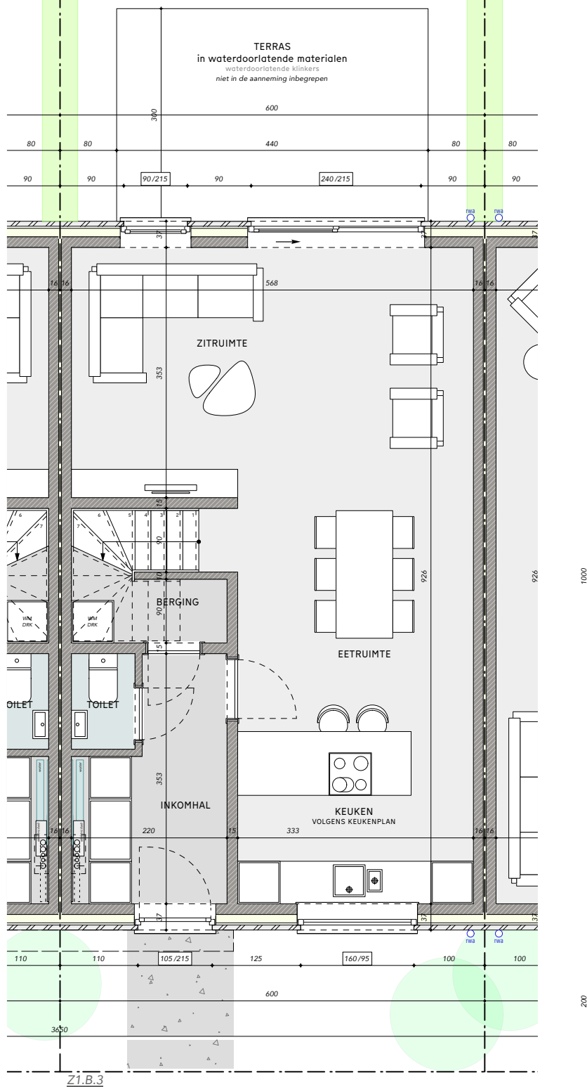
GRONDPLAN gelijkvloers
