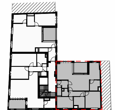
1° verdieping
