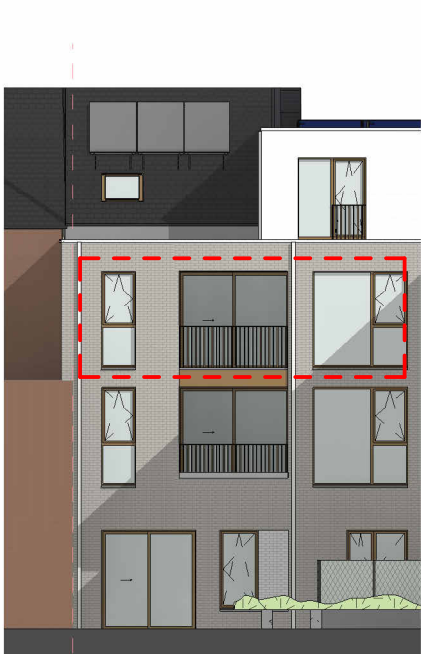
Achtergevel
