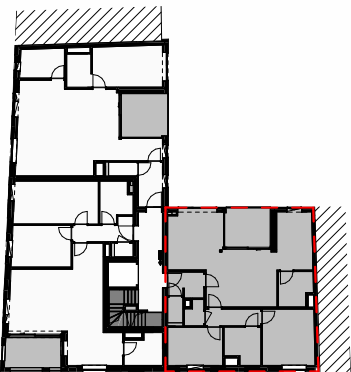
2° verdieping
