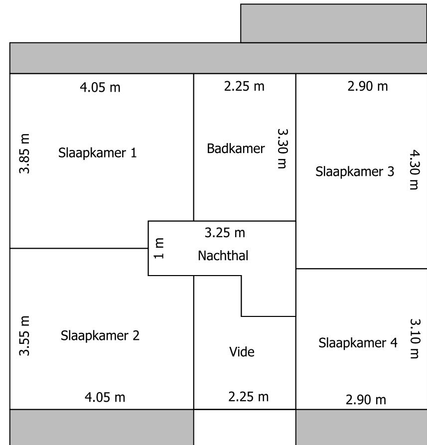
1ste verdieping
