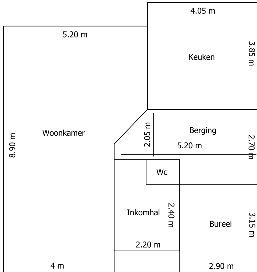
Gelijkvloers
