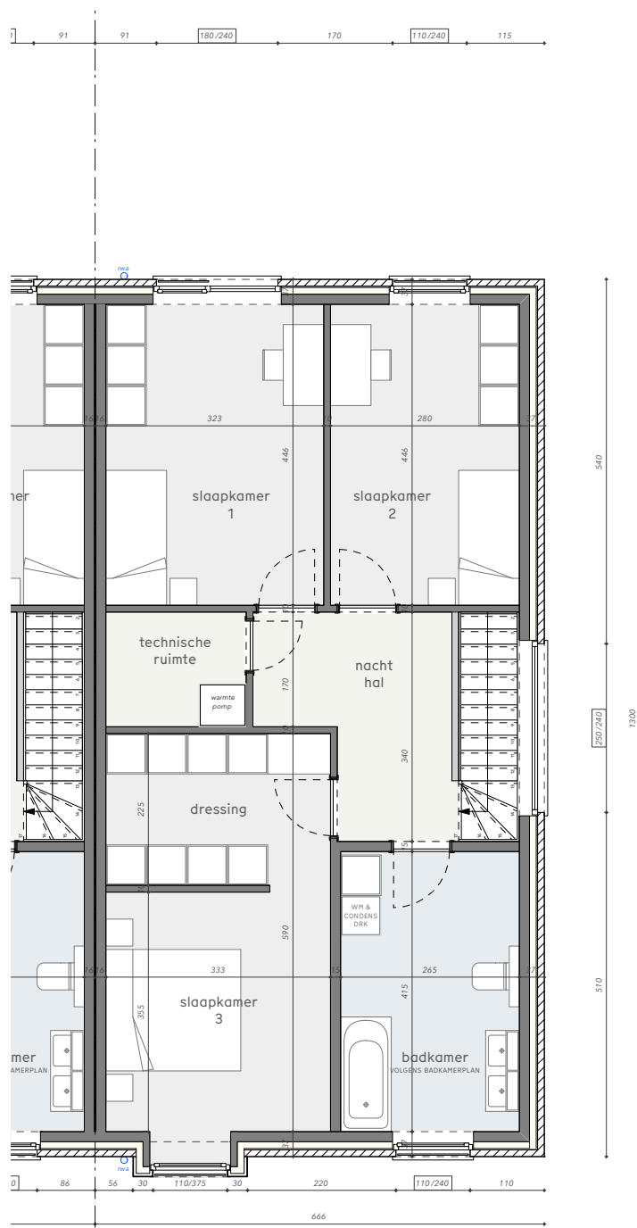
grondplan verdieping
