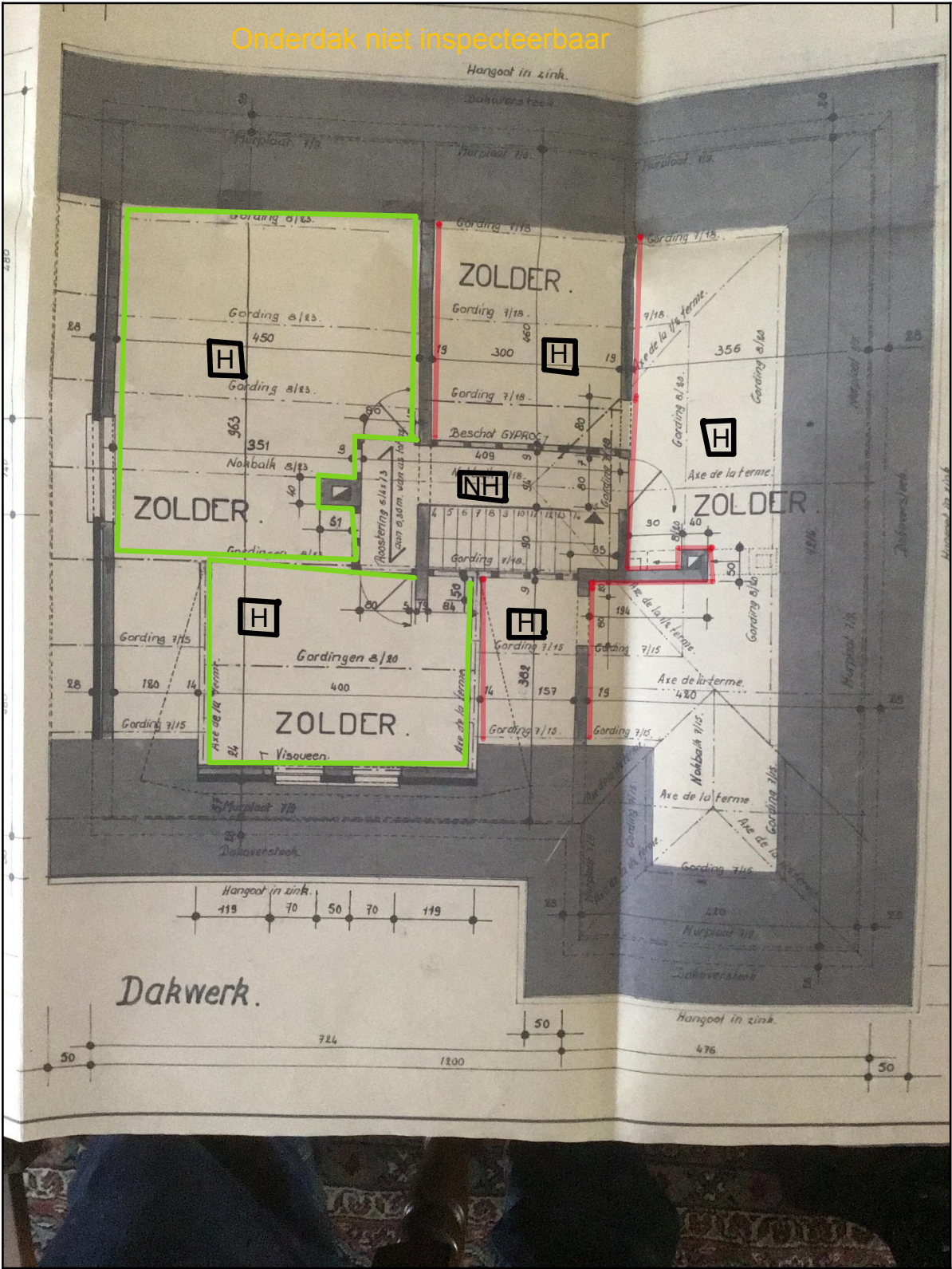
Legende van plan 1.4: Hoofdgebouw plan zolder
