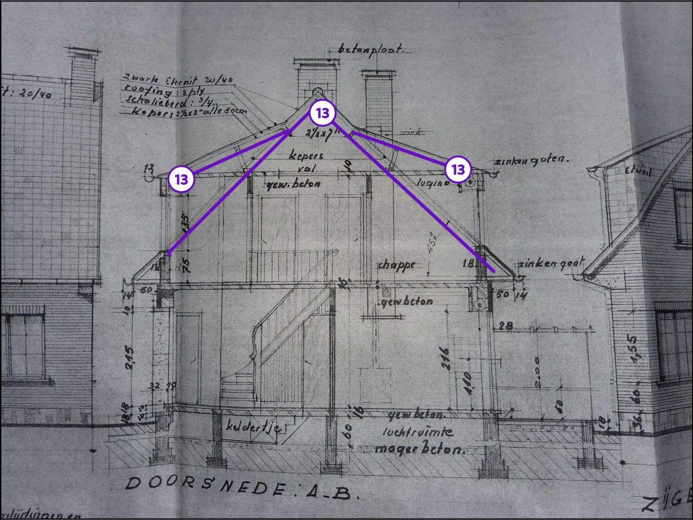
Legende van plan 1.7: Doorsnede
