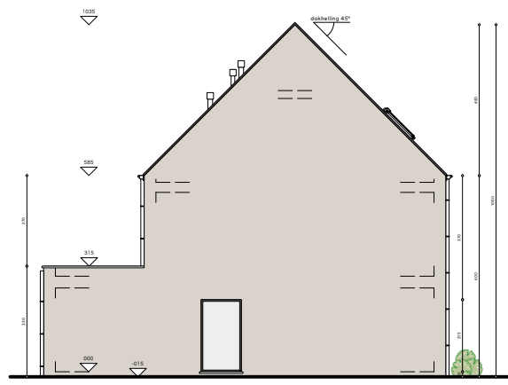
aanzicht zijgevel
