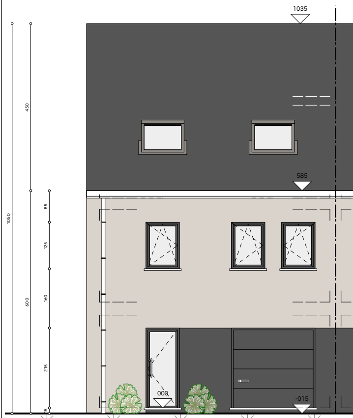
aanzicht voorgevel
