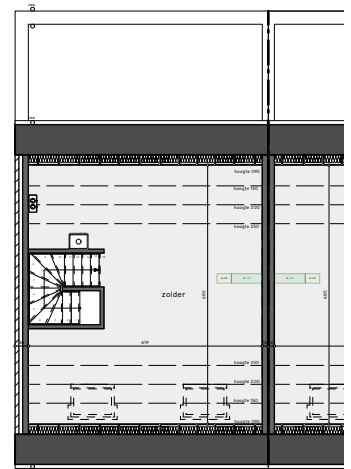
grondplan zolder
