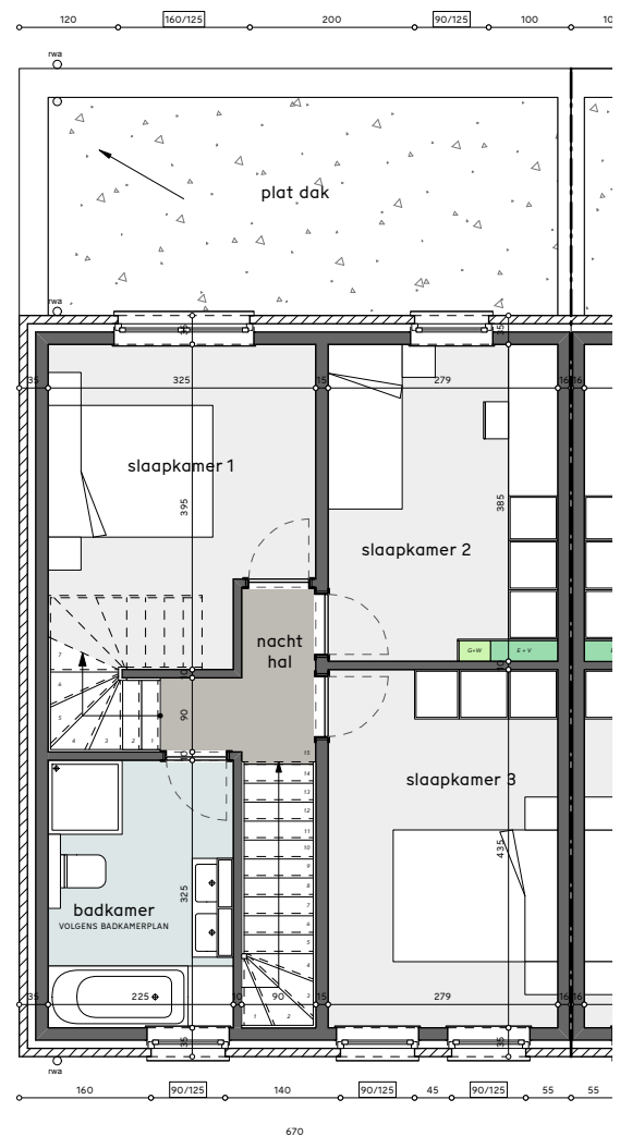
grondplan verdieping
