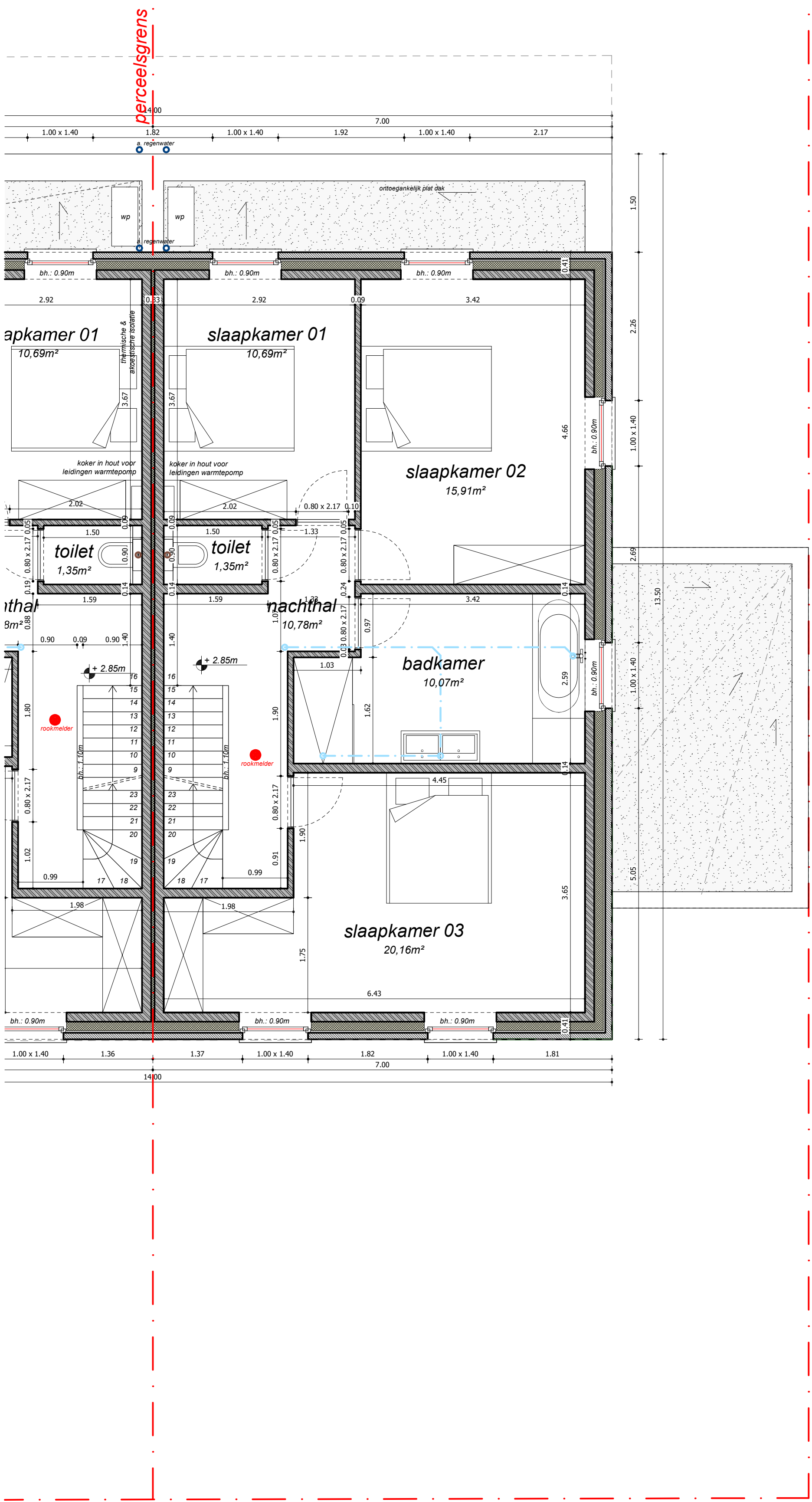
VERDIEPINGSPLAN
