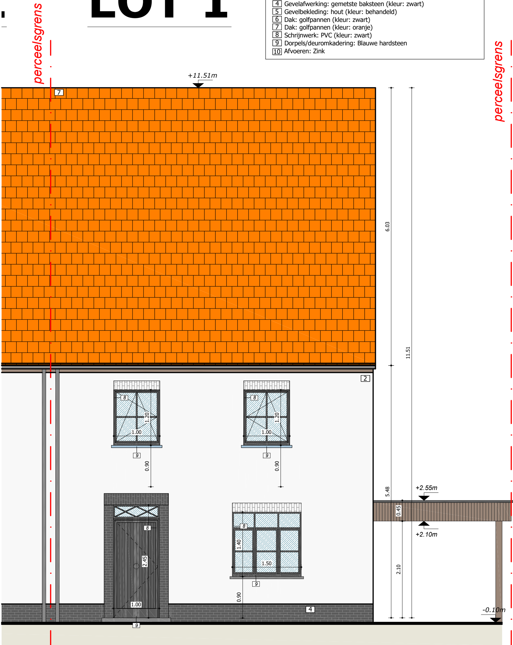
VOORGEVEL SCHAAL 1:50 0 1 2 3 4 5
