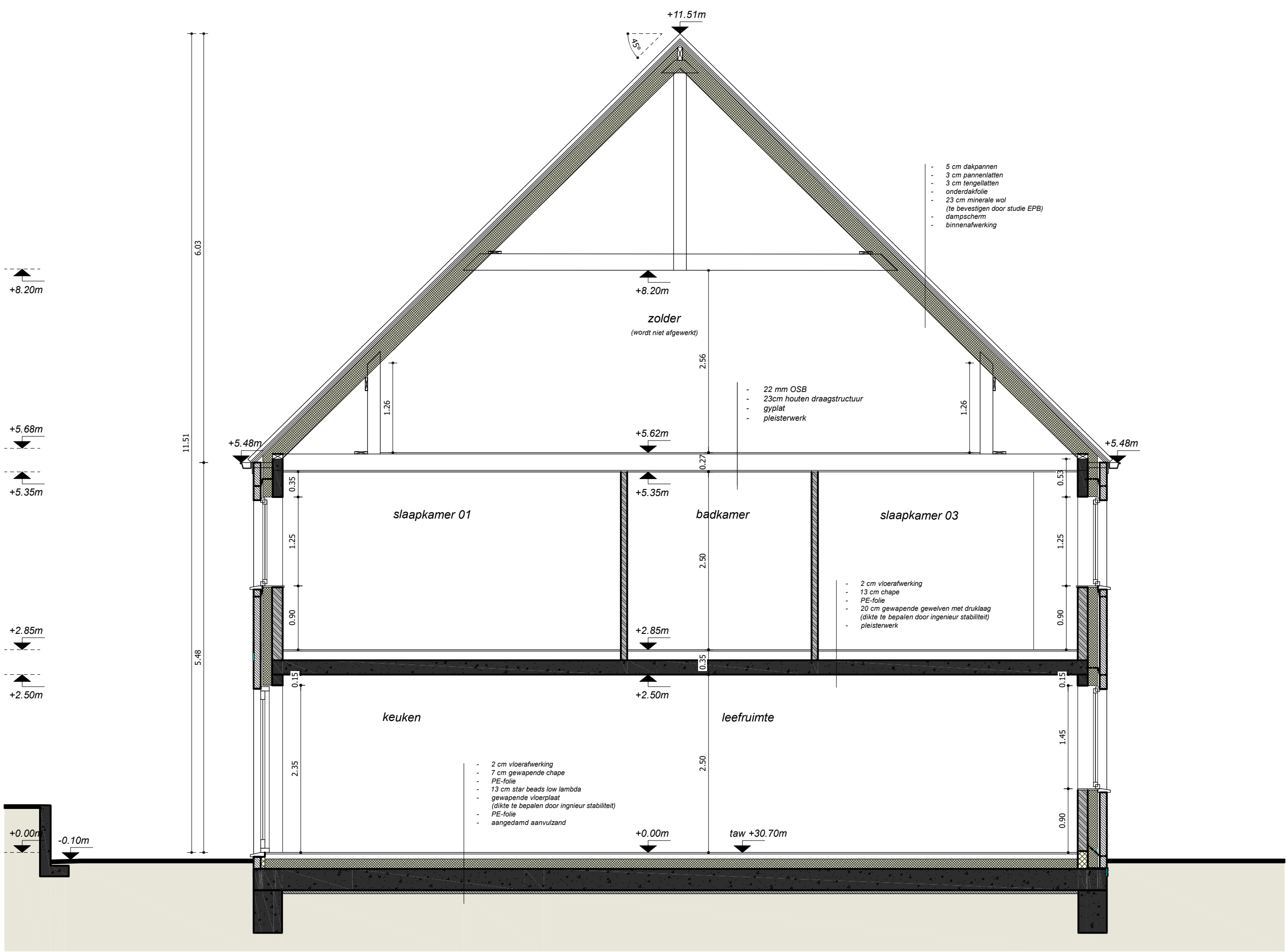
doorsnede GG' schaal 1:50 0 1 2 3 4 5
