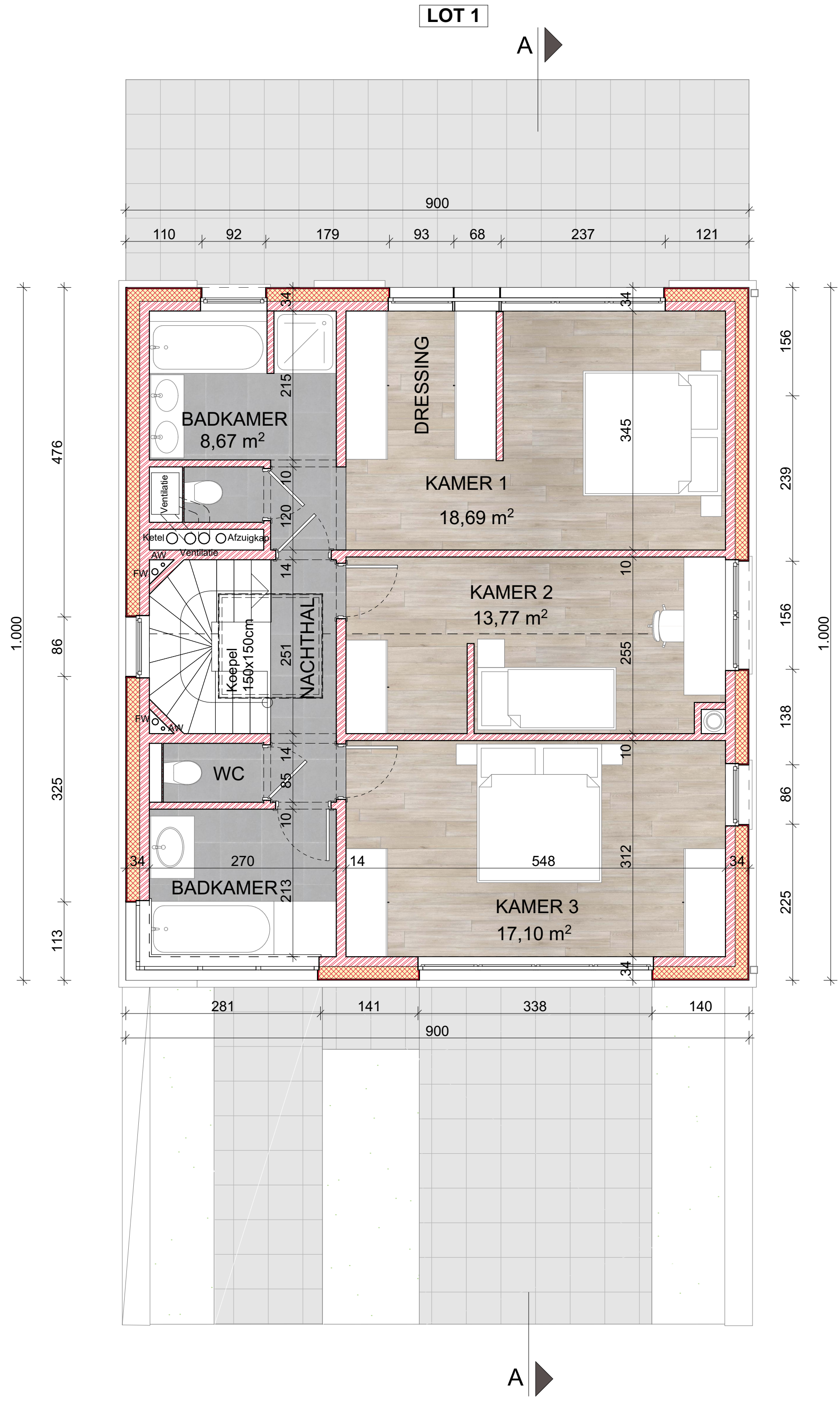
Etage 1 1:50
