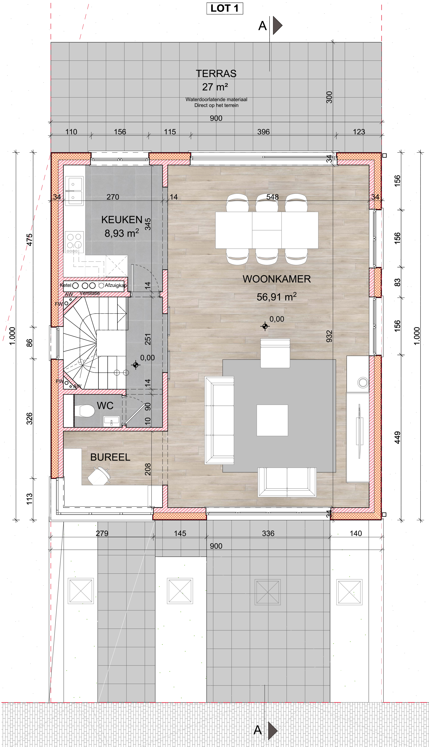
Bel étage 1:50
