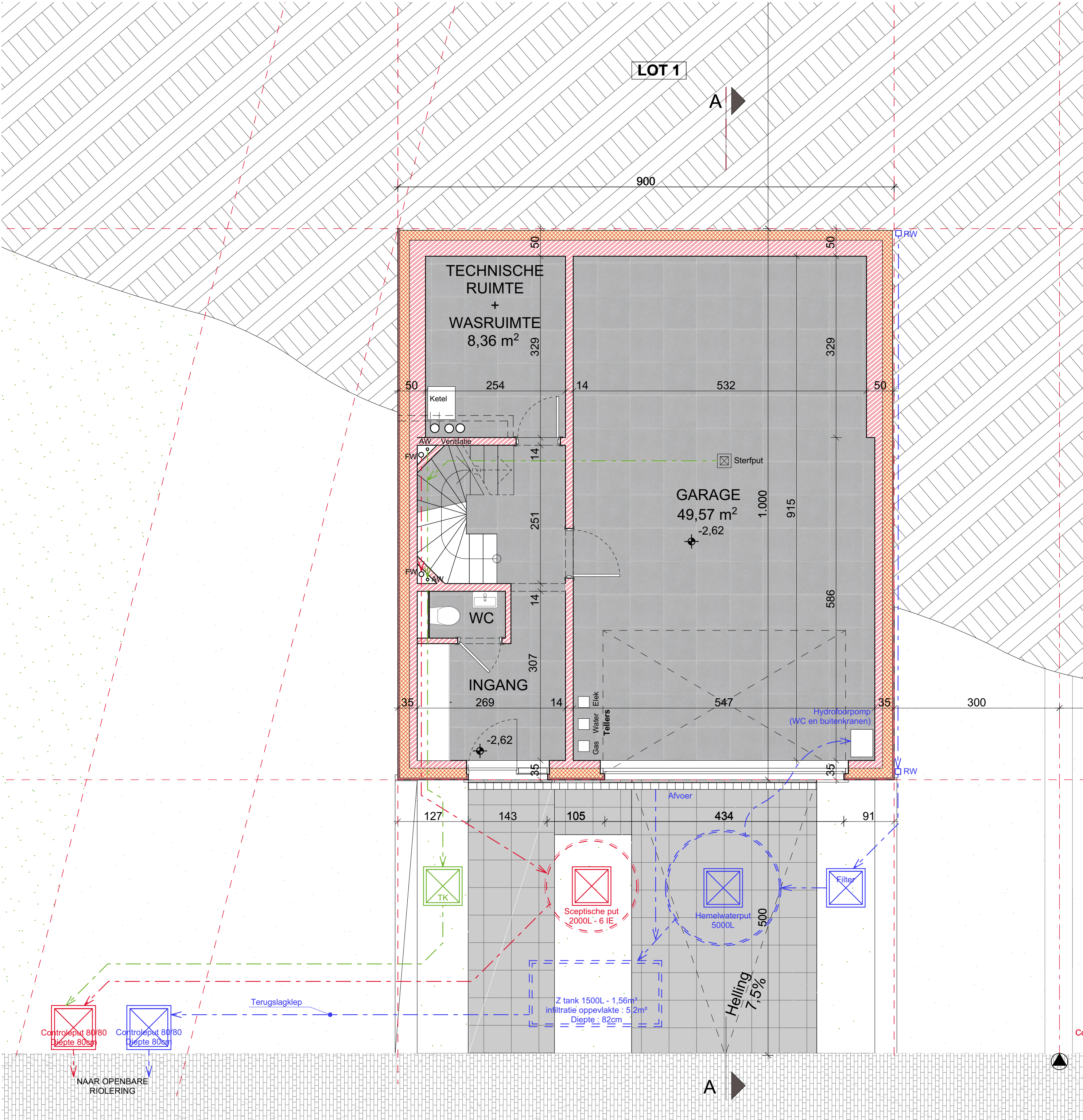
Sous-sol 1:50
