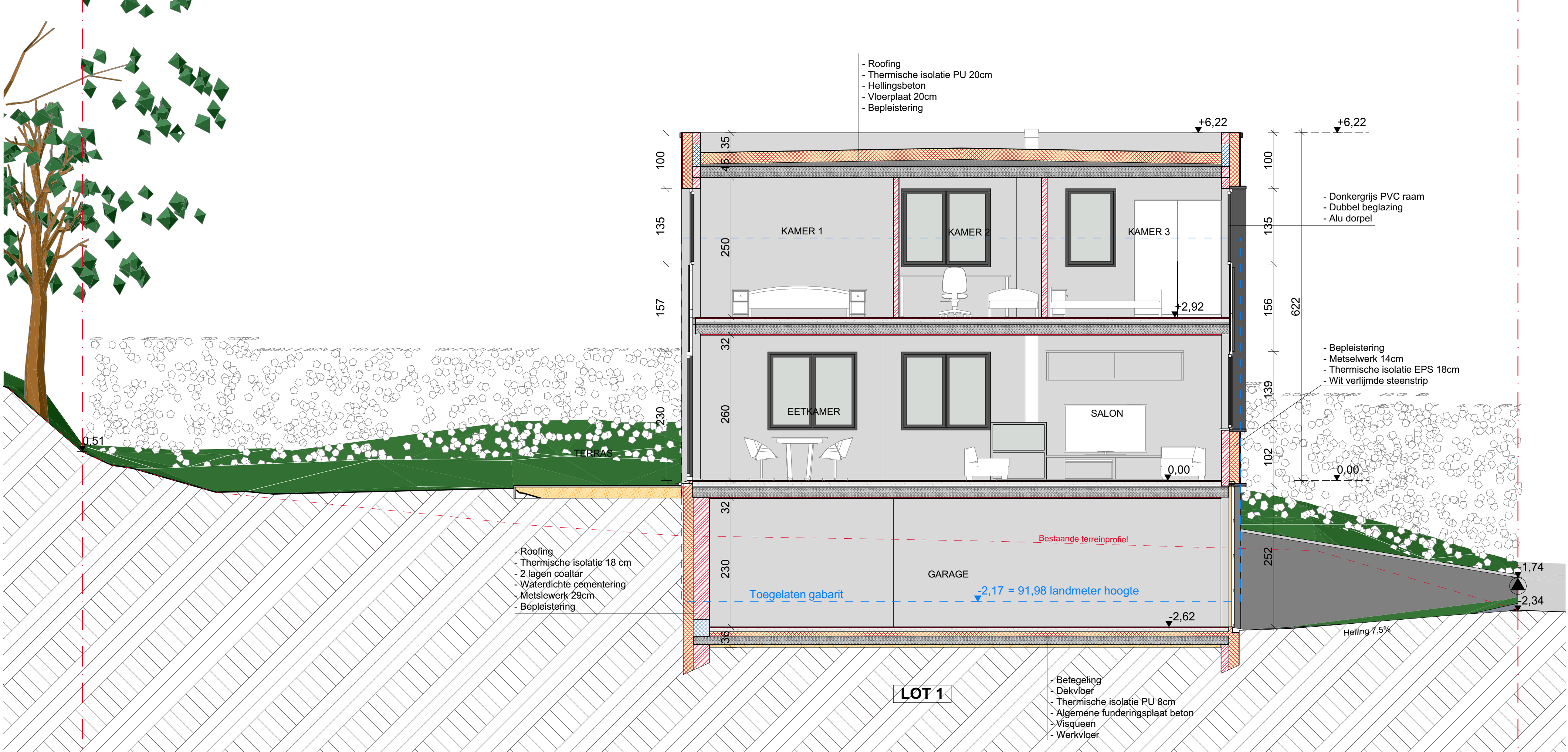
Coupe AA 1:50
