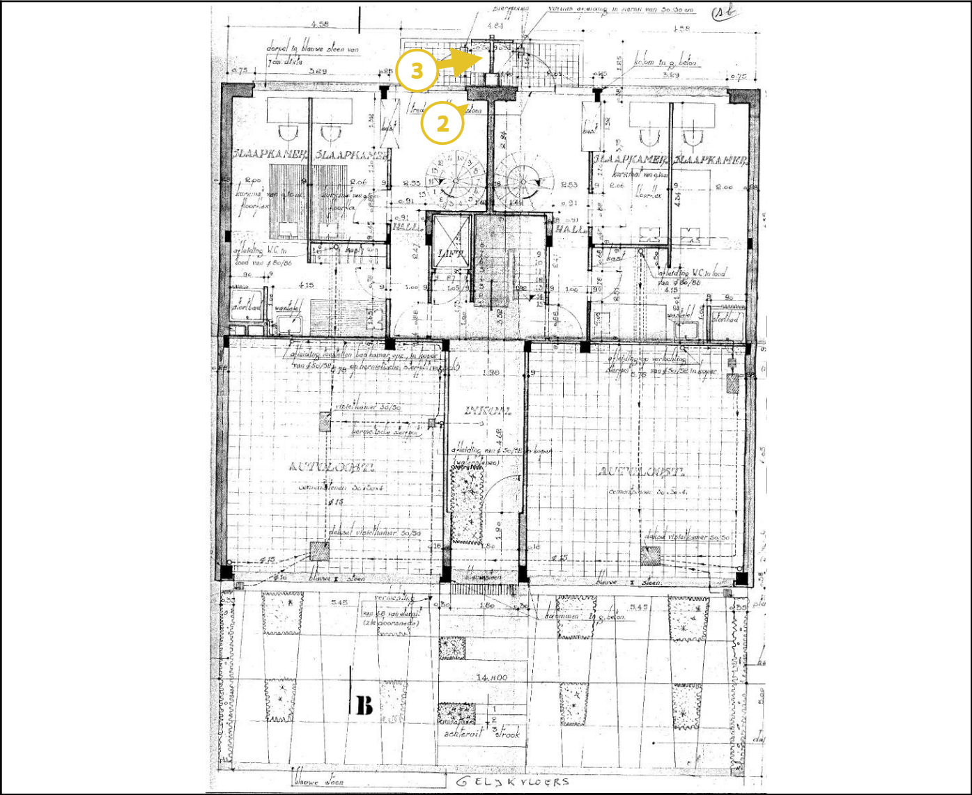
Legende van plan 1.3: gelijksvloer
