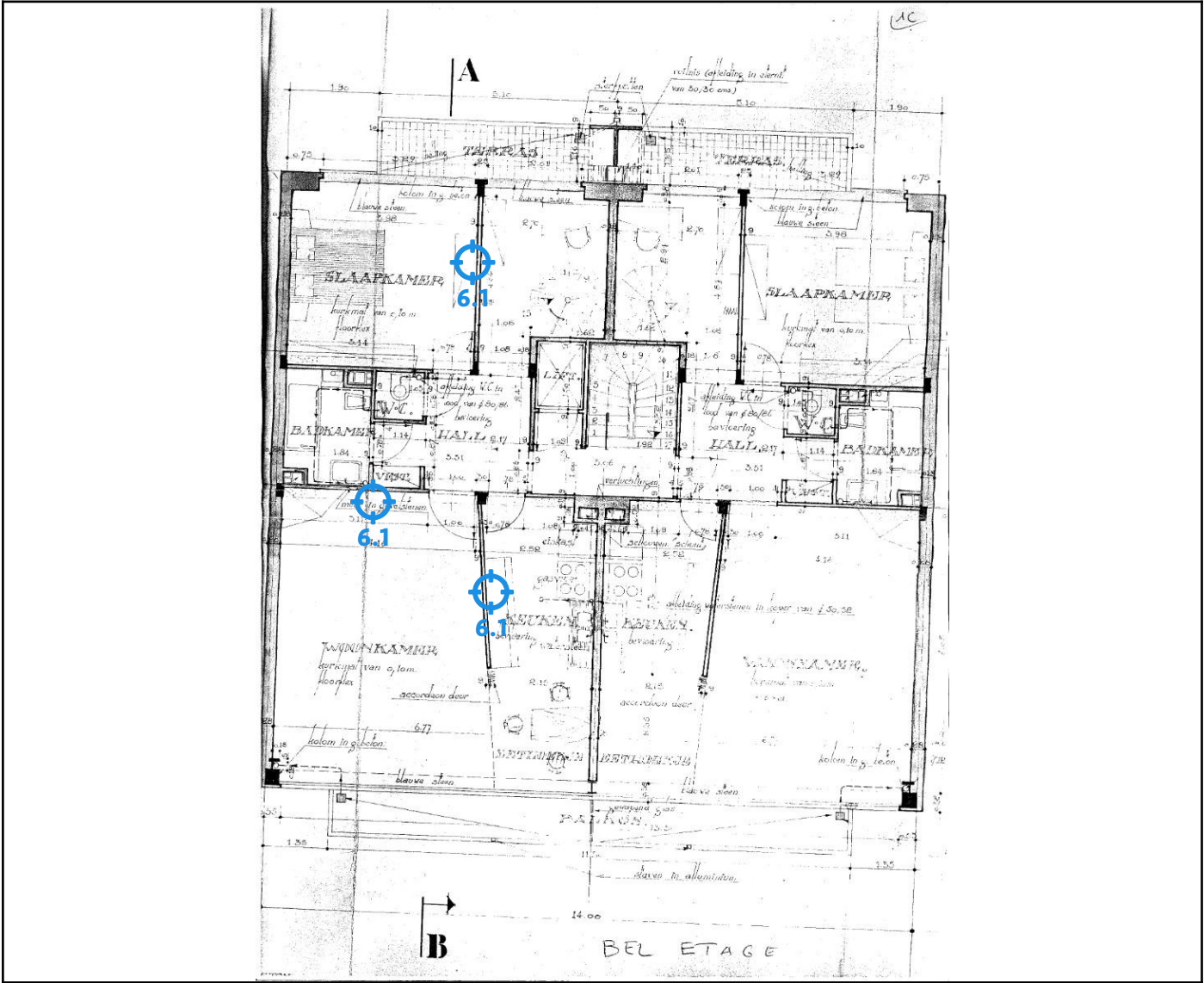
Legende van plan 1.7: 1ste verdiep stalen pleisterwerk muren
