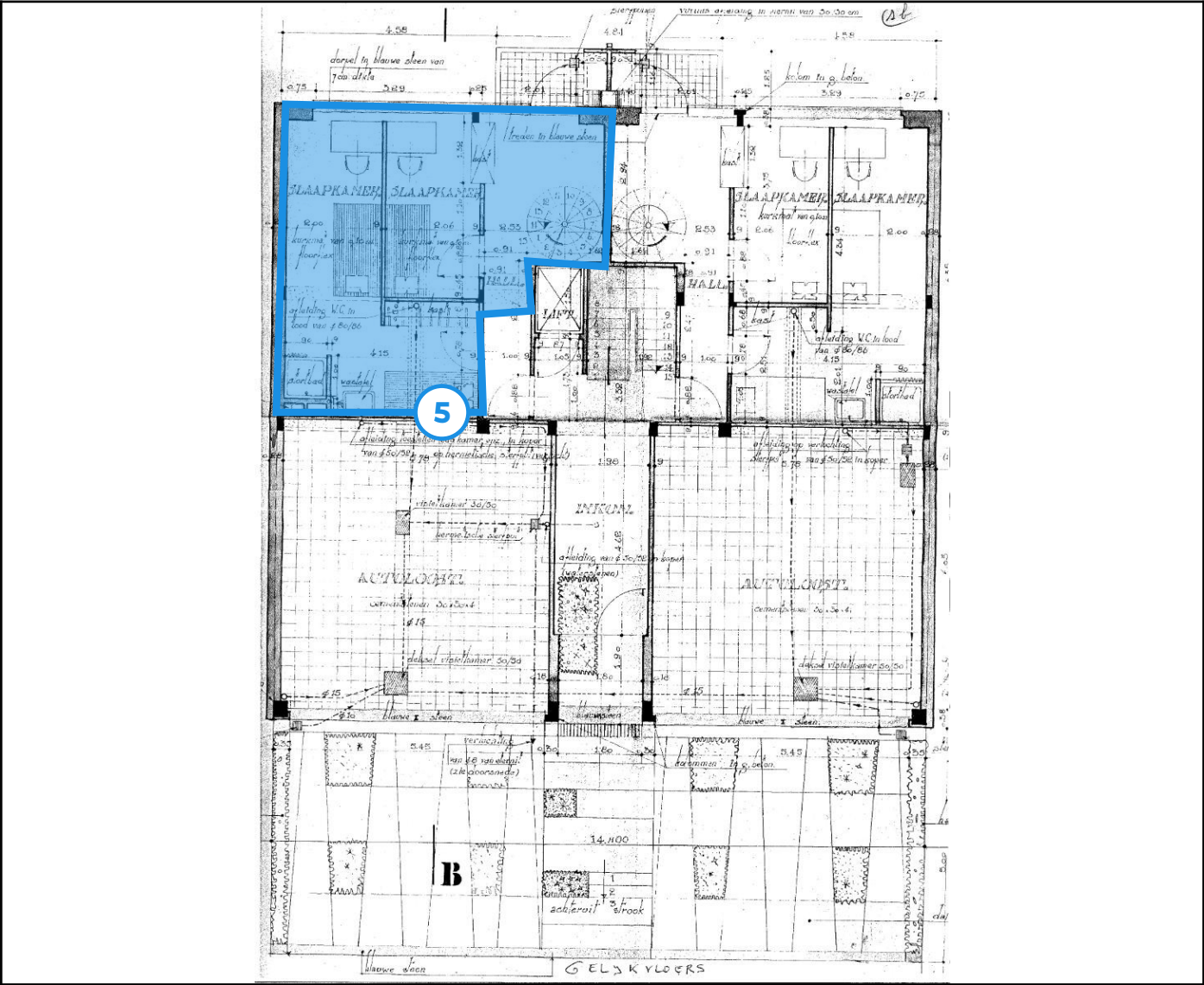
Legende van plan 1.10: gelijkvloer pleister plafond
