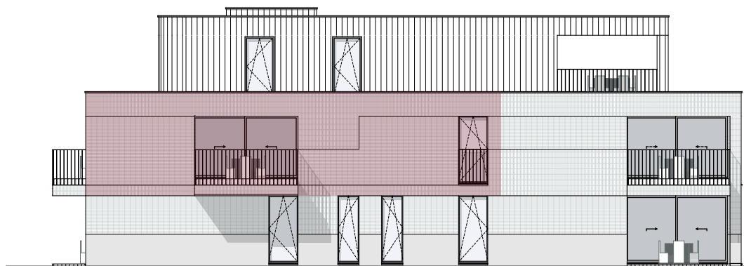
Achtergevel
