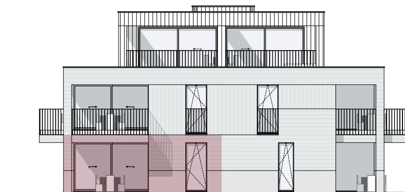
Zijgevel links
