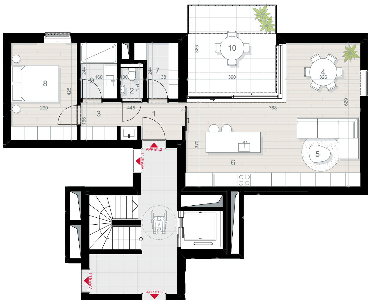
App.B.1.2 | grondplan
