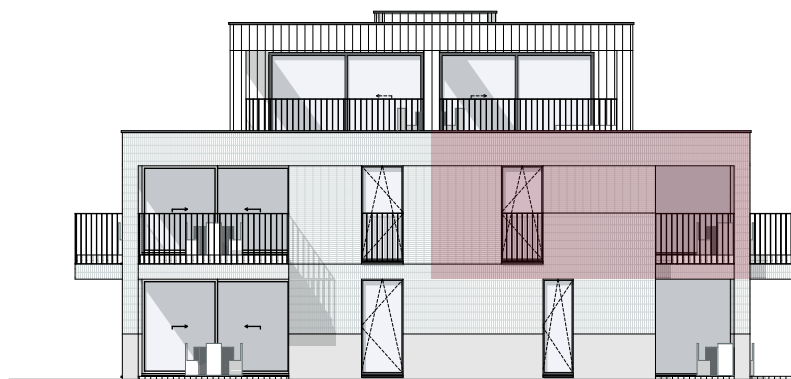
Zijgevel links
