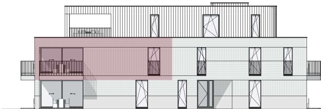
Voorgevel
