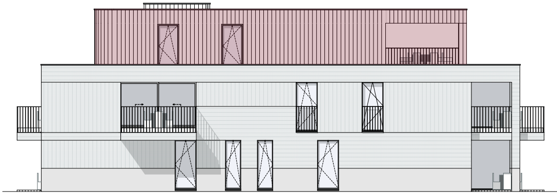
Achtergevel
