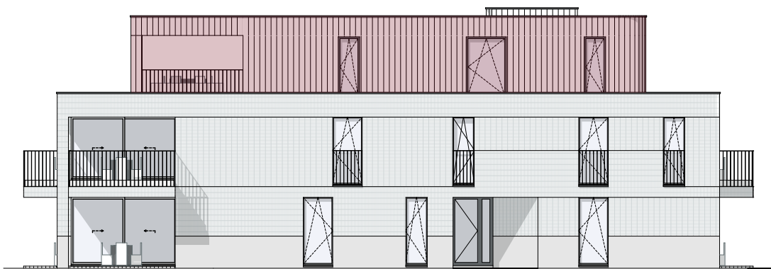
Vorgevel
