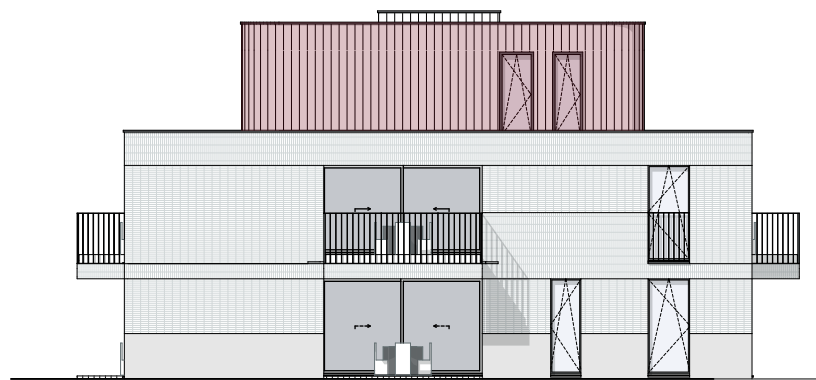
Zijgevel rechts
