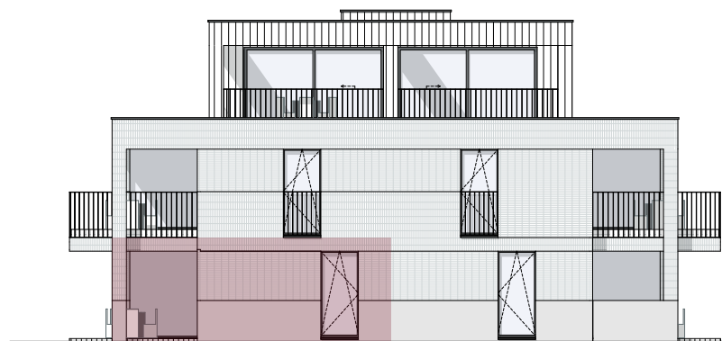
Zijgevel links
