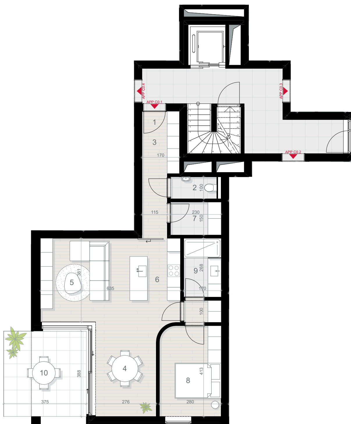
App.C.0.1 | grondplan
