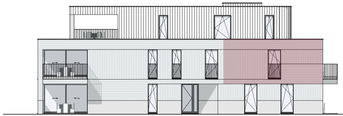
Vorgevel
