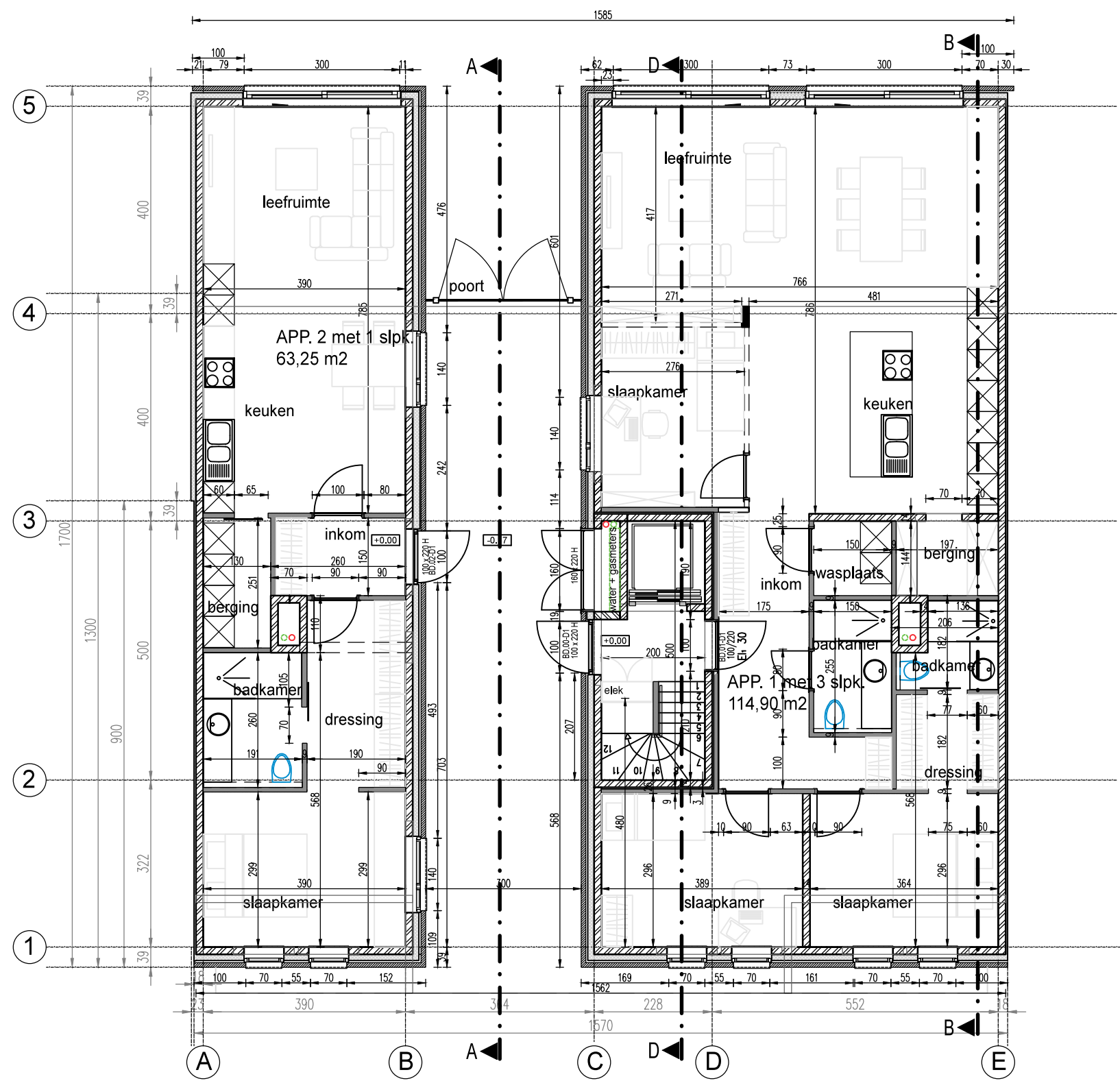
GRONPLAN GELIJKVLOERSE VERDIEPING
