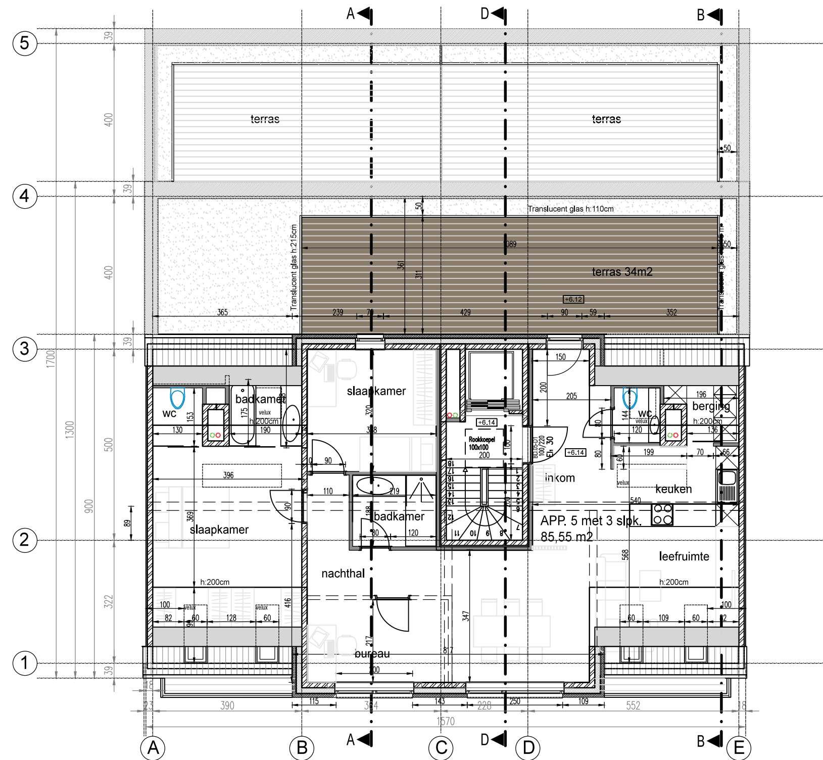
GRONPLAN 2de VERDIEPING
