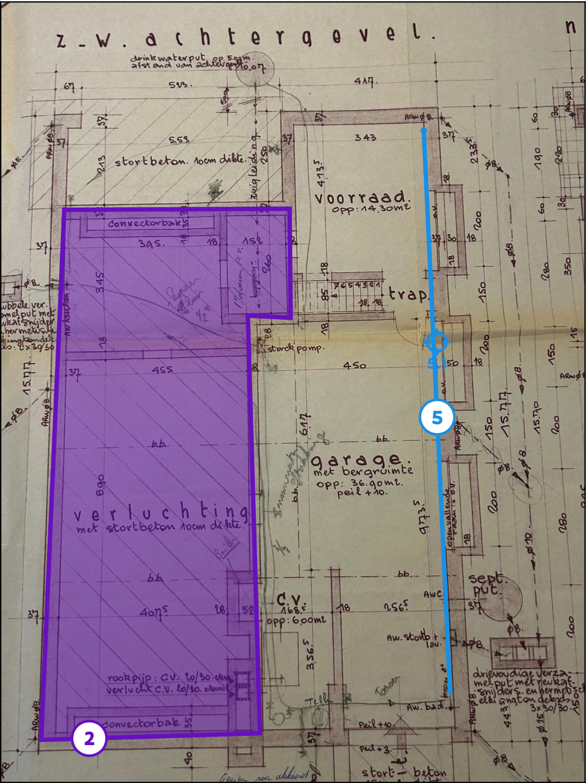
Legende van plan 1.1: Kelder - garage
