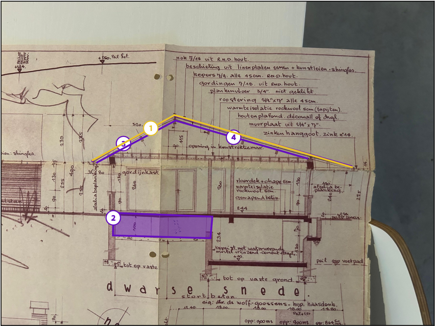
Legende van plan 1.3: Doorsnede
