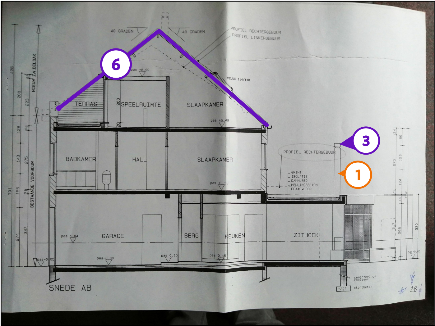
Legende van plan 1.4: snede
