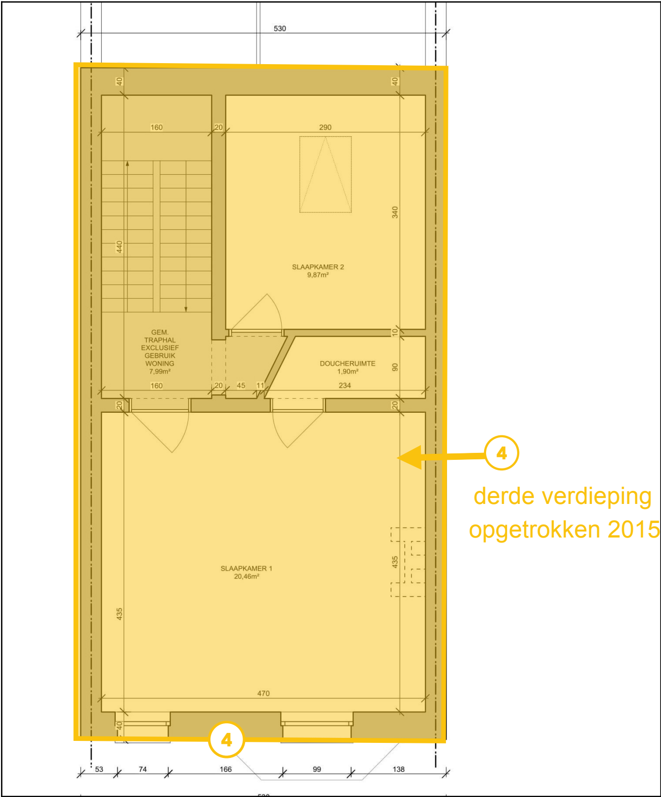
Legende van plan 1.16: Plan verdieping 3 - renovatie en opgetrokken 2015
