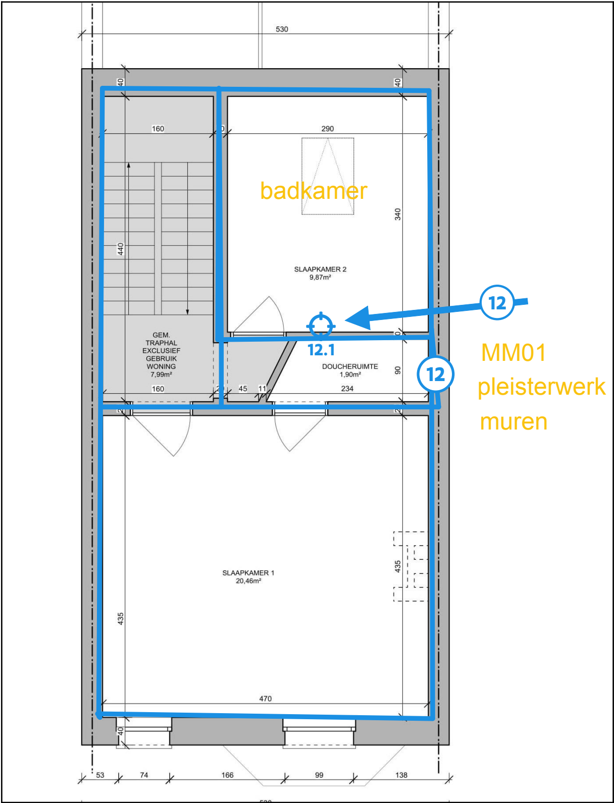
Legende van plan 1.4: Plan verdieping 3 - pleisterwerk muren
