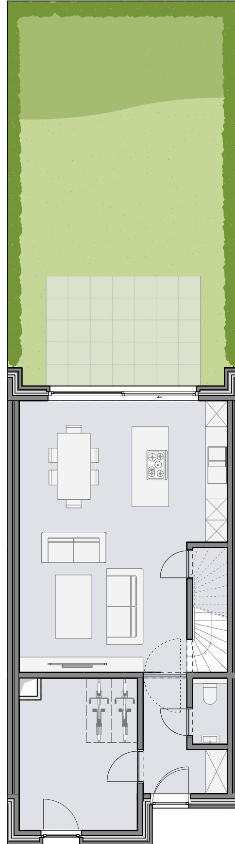
grondplan +00
