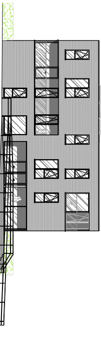
ZIJGEVEL LINKS
