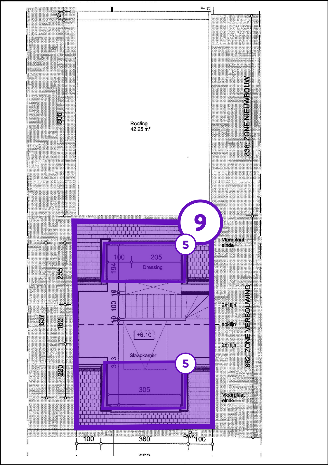
Legende van plan 1.4: grondplan zolderverdiepng
