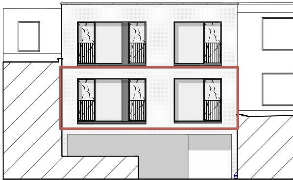
ACHTERGEVEL BINNENGEBIED
